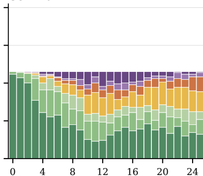
Gemma 2 2B
