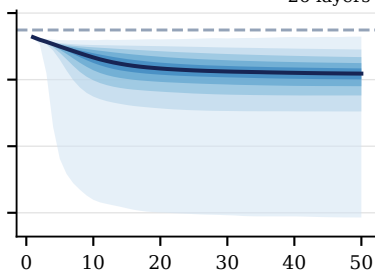
Gemma 2 2B
