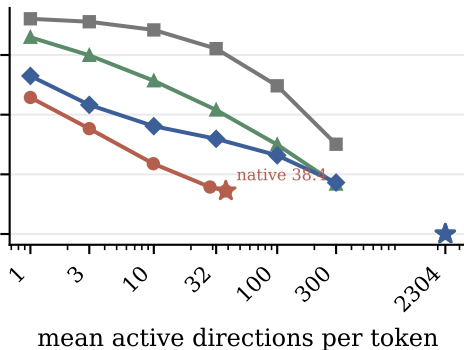
Gemma 2 2B
