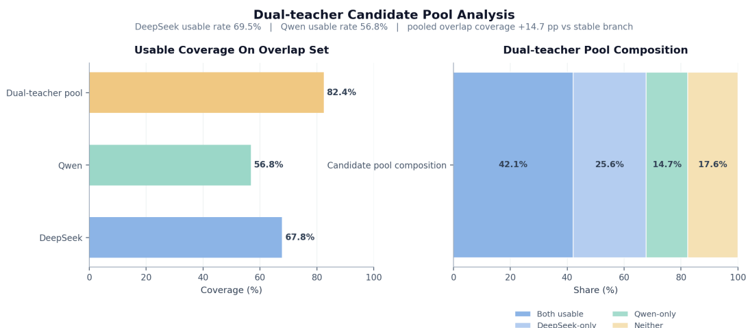
图 6-2 双教师候选池互补性分析：左图为双教师重叠题集上的高纯可用覆盖率，右图为候选池组成占比。双教师并行候选生成可将高纯覆盖率提升至 82.4% ，较稳定教师单支路提高约 14.7 个百分点
