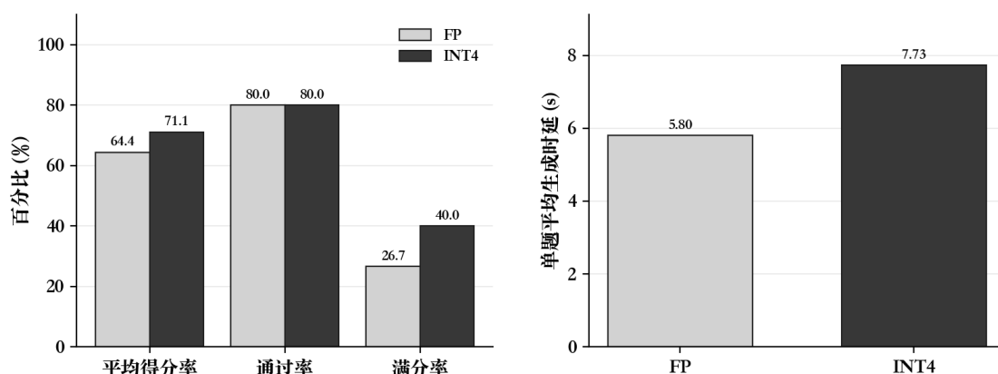
图 7-2 P0.5 本地 FP 与部署版 INT4 对比：左为平均得分率/通过率/满分率，右为单题平均生成时延。
