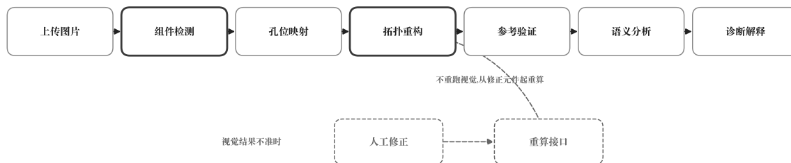
图 2-3 主业务流程：上排为自动诊断主链（上传图片 → 组件检测 → 孔位映射 → 拓扑重构 → 参考验证 → 语义分析 → 诊断解释）；下方为人机协同修正回路——视觉结果不准时，人工修正后从拓扑重构起重算，不重跑视觉检测
