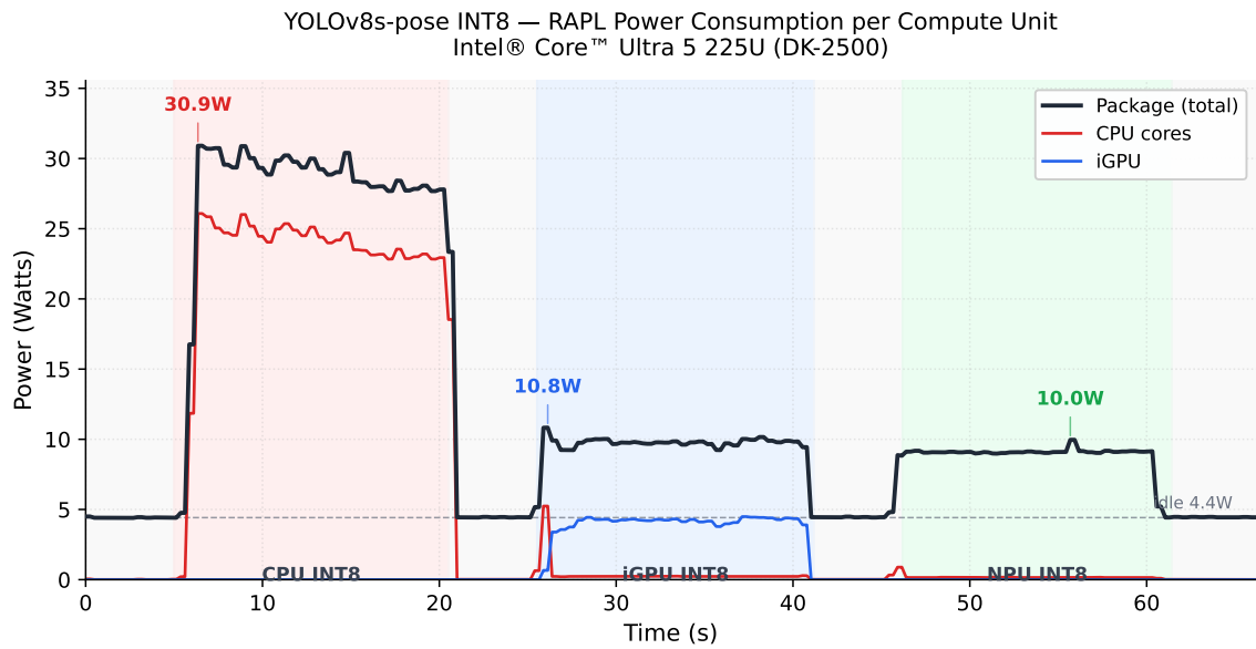
图 7-2 YOLOv8s-pose INT8 在 DK-2500 上的 RAPL 功耗时序（turbostat 0.25 s 采样）。横轴为时间，纵轴为瓦特；颜色分别为 Package 总功率（黑）、CPU cores（红）、iGPU（蓝）。三段彩色背景对应 CPU/iGPU/NPU 三种 worker 各自 sustained 15 秒的工作态，期间生成 498/841/1153 次推理。CPU 工作态峰值 30.9 W，几乎全部由 CPU cores 承担；iGPU 工作态总功率 10.8 W，其中 GFX 4.4 W；NPU 工作态总功率 10.0 W，但 CPU cores 与 GFX 线全程趴在 0——意味着 NPU 推理几乎不占用 CPU/iGPU 资源，是实现真正异构并行的关键。
