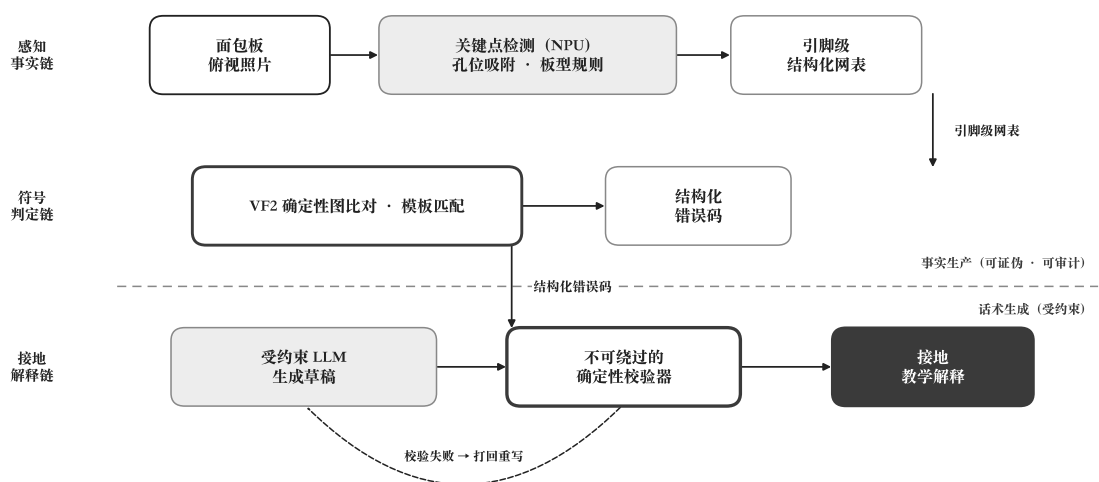
图 2-1 神经—符号解耦的三链路：感知、符号两链“生产”可审计的结构化事实，安全敏感的对错判定只发生在符号判定链（VF2 确定性图比对）；以“事实生产 / 话术生成”为解耦边界，第三链才由受约束小模型把事实改写为教学语言，并经不可绕过的校验器拦截无依据陈述（校验失败即打回重写）
