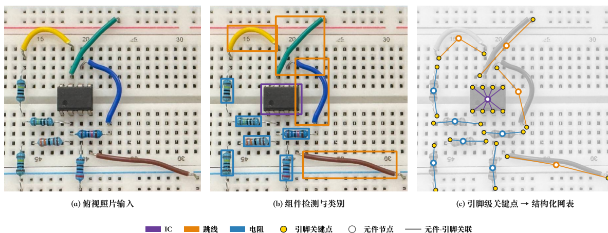
图 4-2 视觉事实链端到端示例（真实模型输出，板上实拍）：(a) 俯视照片输入；(b) 组件检测与类别框；(c) 引脚级关键点汇聚为结构化网表（元件—引脚关联图，IC 引脚按 DIP 封装几何派生）——“像素 → 神经感知 → 符号化结构事实”端到端贯通
