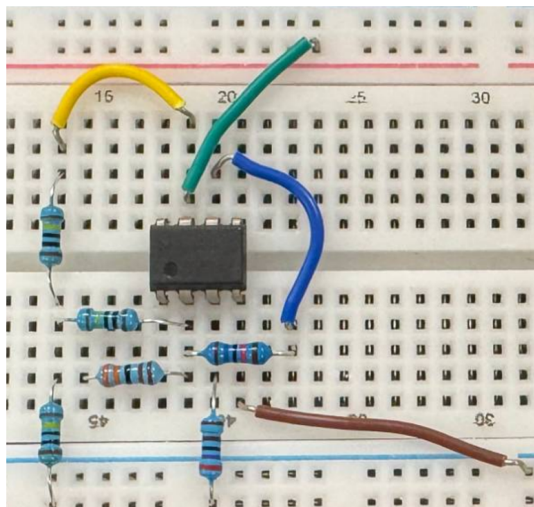
(a) 俯视照片输入
