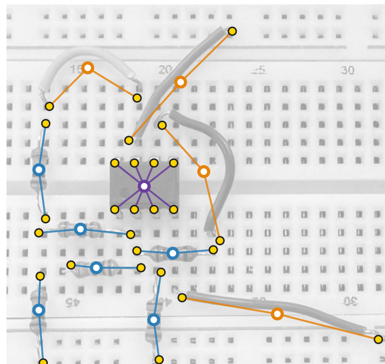
(c) 引脚级关键点 → 结构化网表
