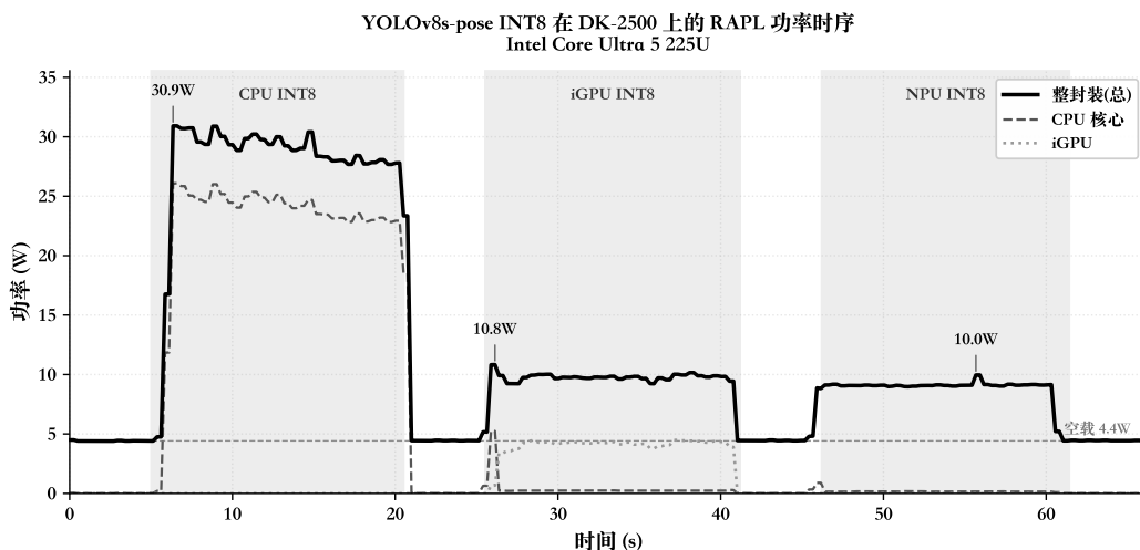
图 6-1 YOLOv8s-pose INT8 在 DK-2500 上的 RAPL 功耗时序：三段分别对应 CPU/iGPU/NPU 各持续 15 秒的工作态；NPU 工作时 CPU 与 iGPU 全程贴近空闲基线，是实现真正异构并行的关键
