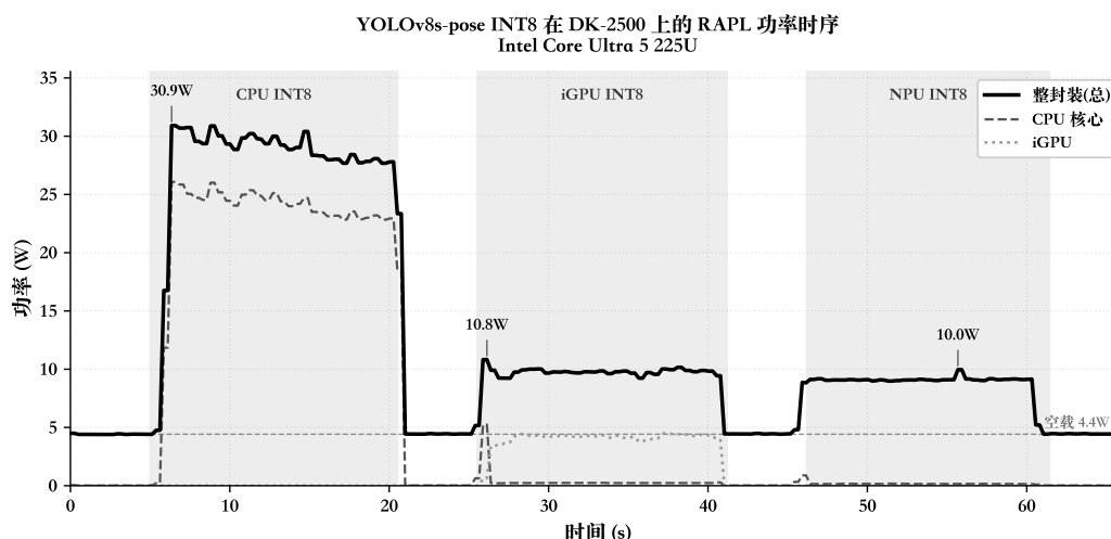
图 6-1 YOLOv8s-pose INT8 在 DK-2500 上的 RAPL 功耗时序：三段分别对应 CPU/iGPU/NPU 各持续 15 秒的工作态；NPU 工作时 CPU 与 iGPU 全程贴近空闲基线，是实现真正异构并行的关键
