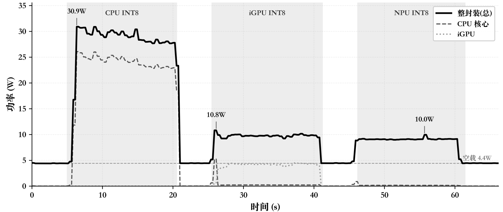
YOLOv8s-pose INT8 在 DK-2500 上的 RAPL 功率时序 Intel Core Ultra 5 225U
