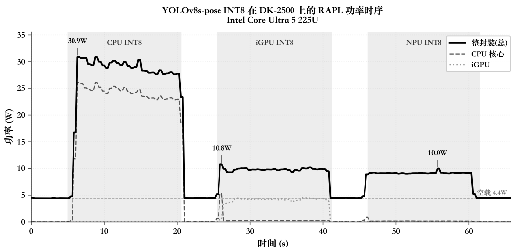
图 6-1 YOLOv8s-pose INT8 在 DK-2500 上的 RAPL 功耗时序：三段分别对应 CPU/iGPU/NPU 各持续 15 秒的工作态；NPU 工作时 CPU 与 iGPU 全程贴近空闲基线，是三单元异构分工、互不争用的硬件前提
