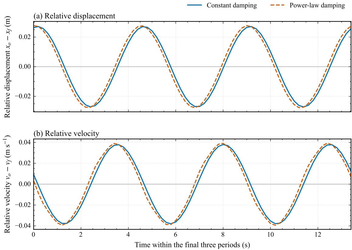
图 4 第 38–40 周期内两种阻尼规律的相对运动对比
