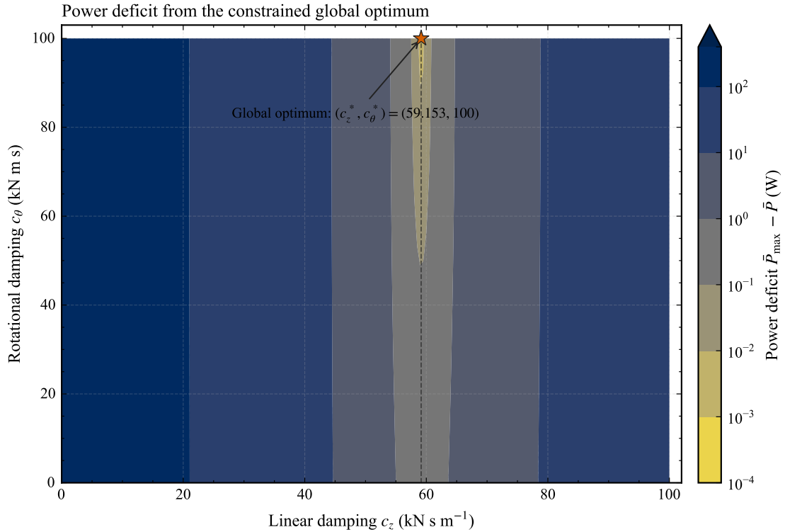
图 12 联合阻尼参数域内相对约束全局最优点的平均功率损失
