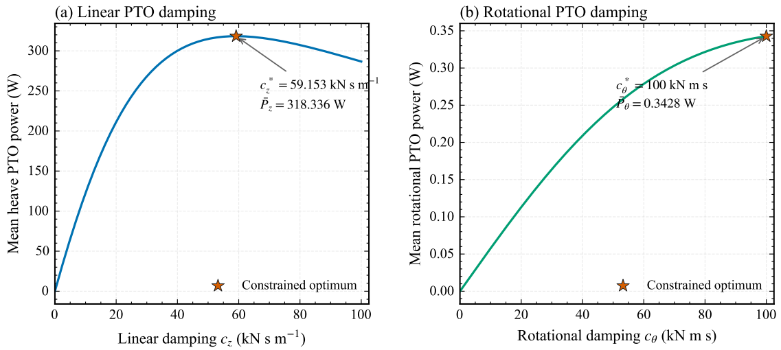
图 11 直线与旋转 PTO 常量阻尼的周期稳态平均功率曲线
