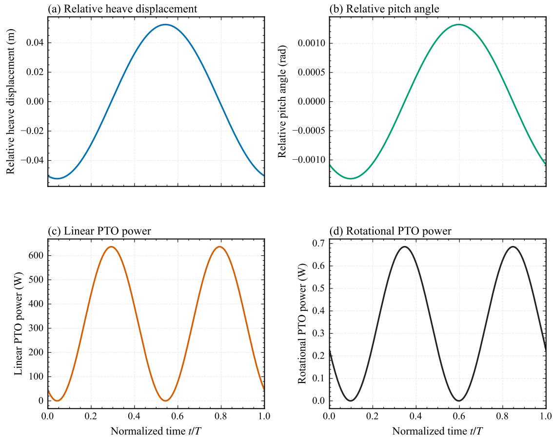
图 13 最优阻尼参数下一个稳定波浪周期的相对运动与 PTO 瞬时功率
