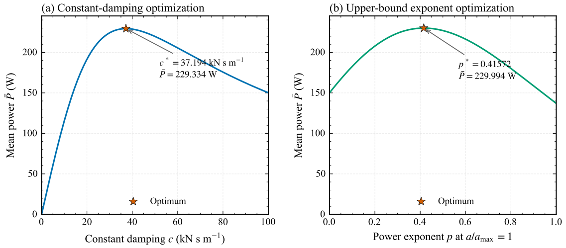
图 6 两类 PTO 阻尼的周期稳态平均功率优化曲线
