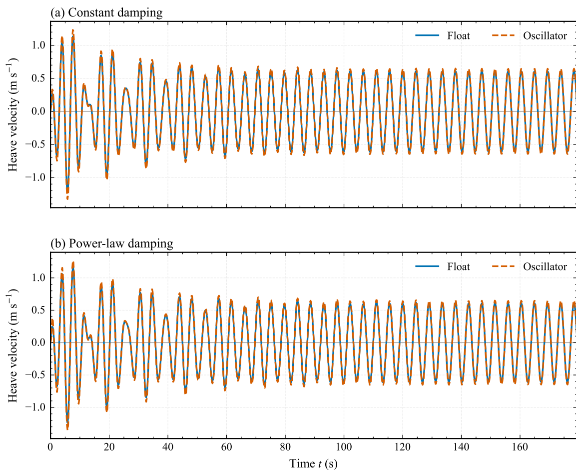
图 3 两种阻尼规律下浮子与振子的垂荡速度响应
