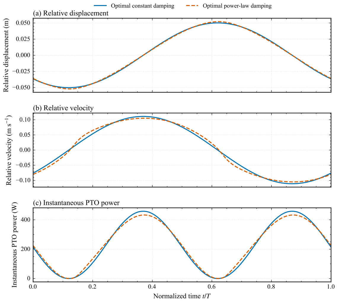
图 7 两种最优 PTO 阻尼下一个稳定周期的响应与输出功率
