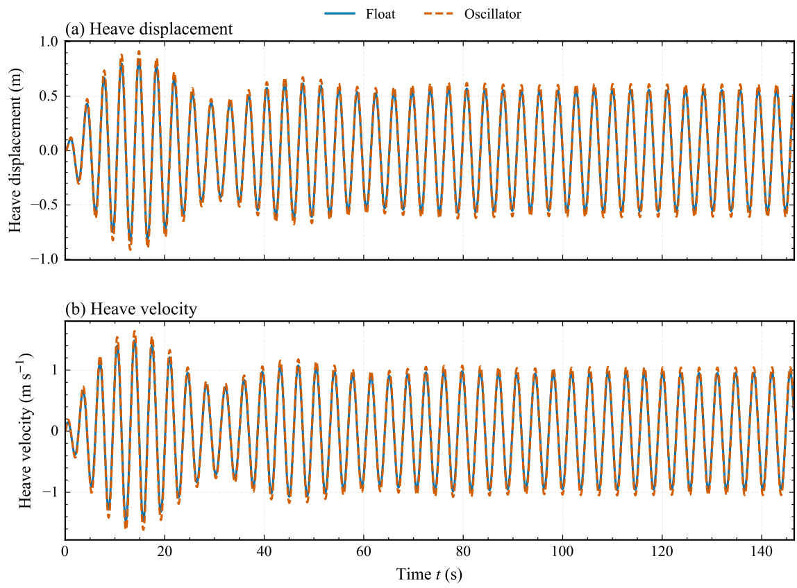
图 8 情形 3 下浮子与振子的垂荡位移和速度响应
