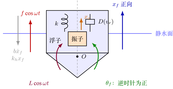
图 1 浮子-振子系统的坐标、PTO 连接与受力示意
