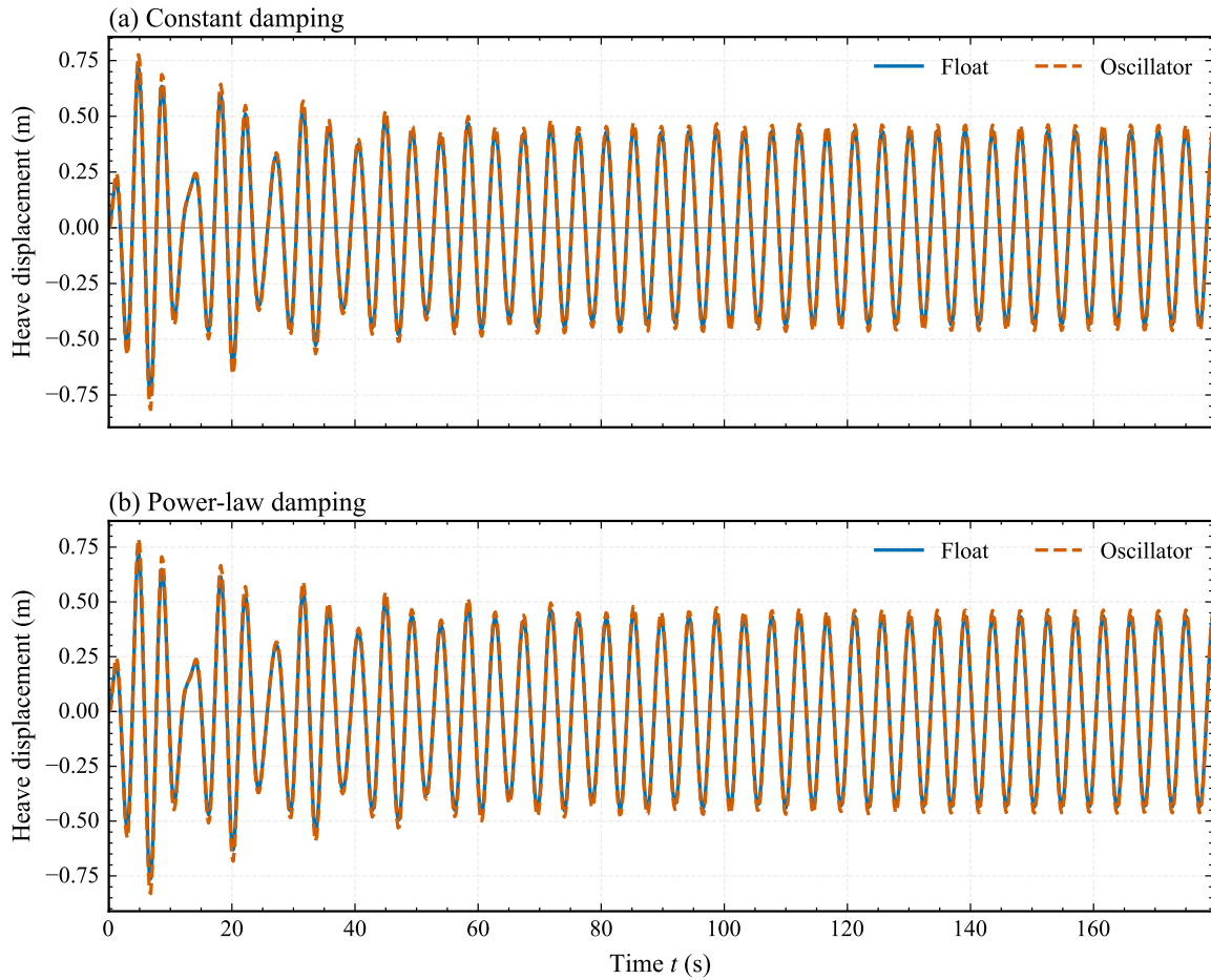
图 2 两种阻尼规律下浮子与振子的垂荡位移响应
