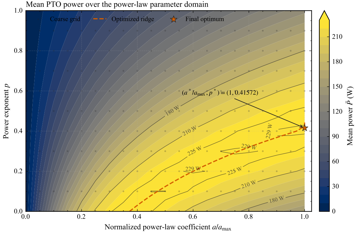
图 5 归一化幂律阻尼参数域内的周期稳态平均功率与高功率脊线
