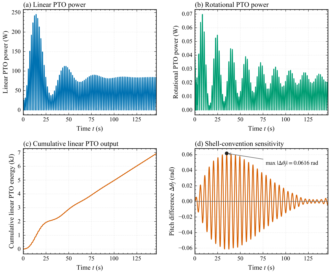
图 10 两类 PTO 输出与浮子壳体口径敏感性
