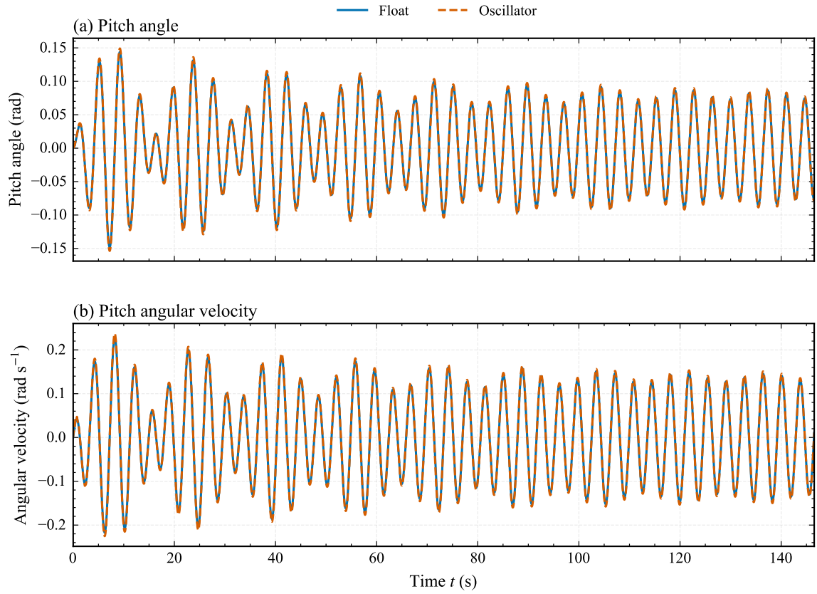
图 9 情形 3 下浮子与振子的纵摇角和角速度响应
