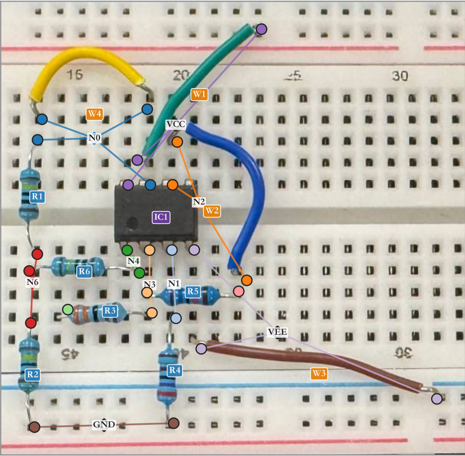
(a) 重构网表 · 面包板视图 (同色 = 同一电气节点)
