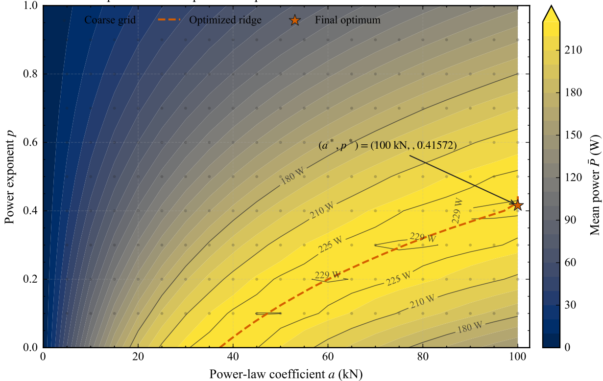
Mean PTO power over the power-law parameter domain
