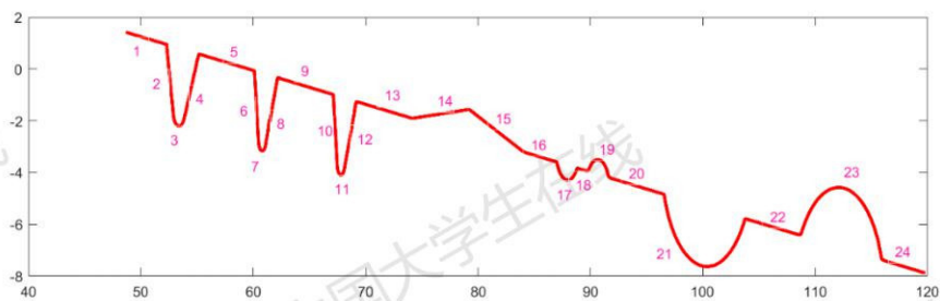
图 5.2.1-1 工件一倾斜并位移后的轮廓
