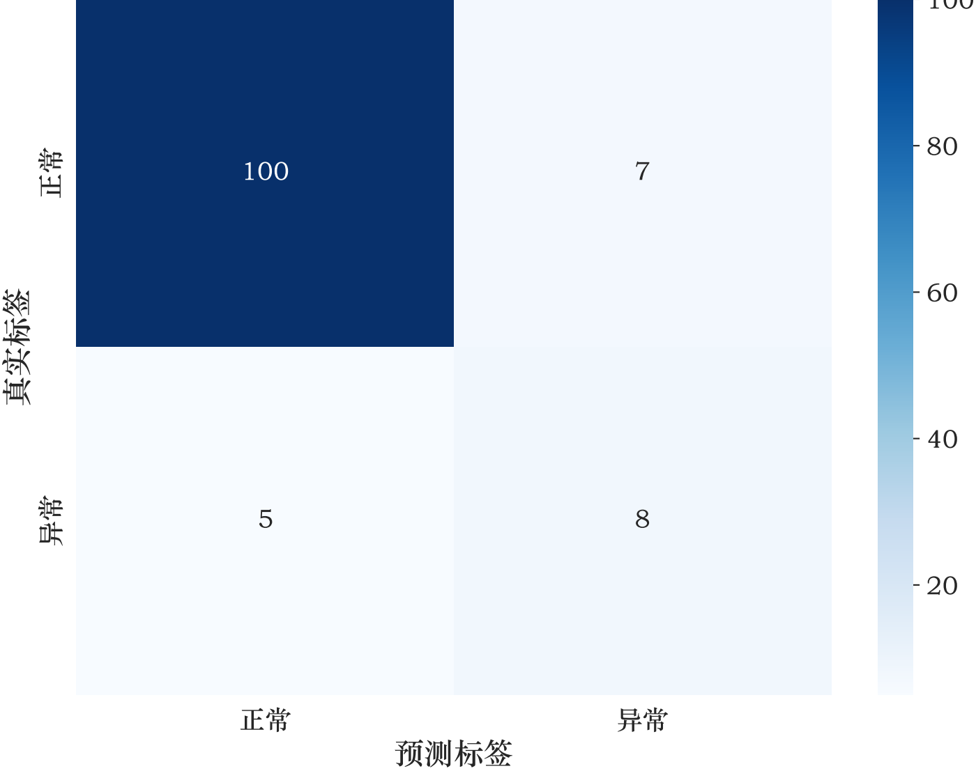
SMOTETomek数据集混淆矩阵
