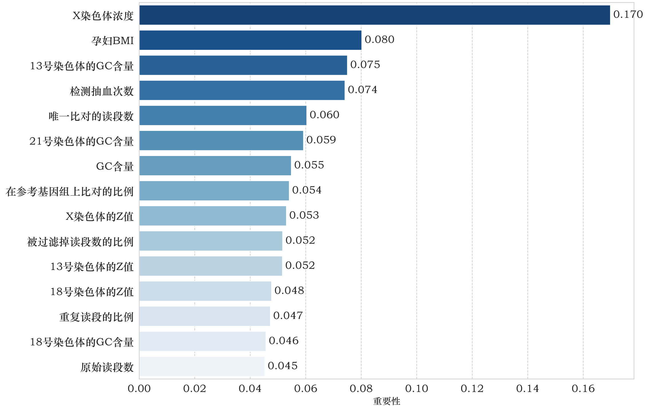
特征重要性排序（前15个）
