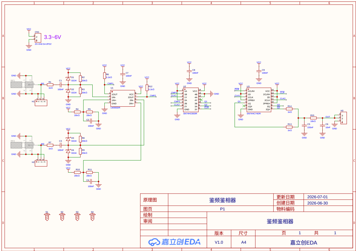
图 3 鉴频鉴相器与鉴相低通输出原理图
