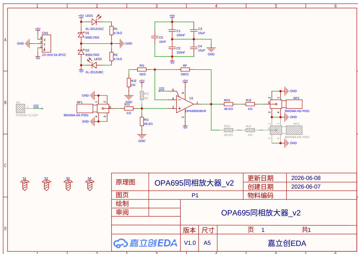
图 4 OPA695 同相放大器与输出调理原理图
