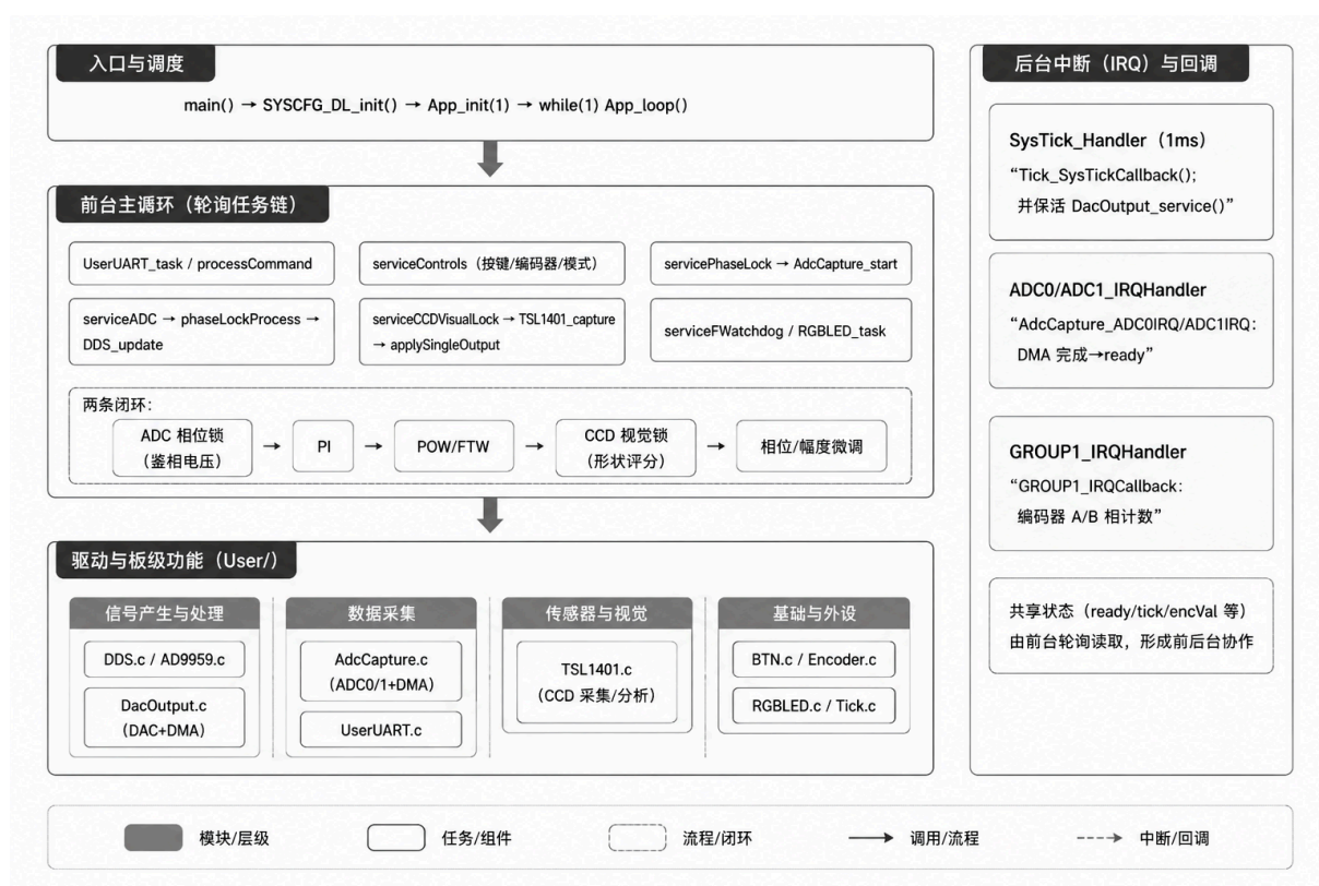
图 5 固件软件架构与前后台协作框图
