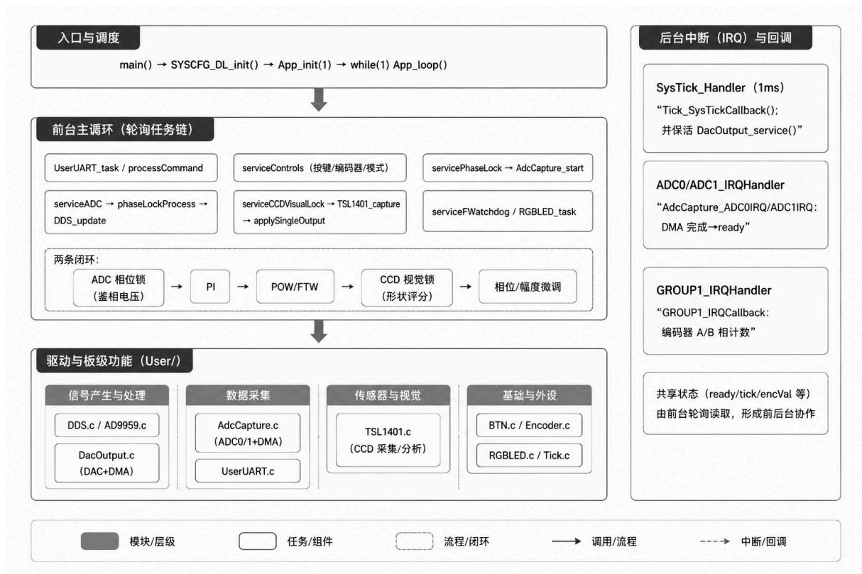
图 2 固件软件架构与前后台协作框图
