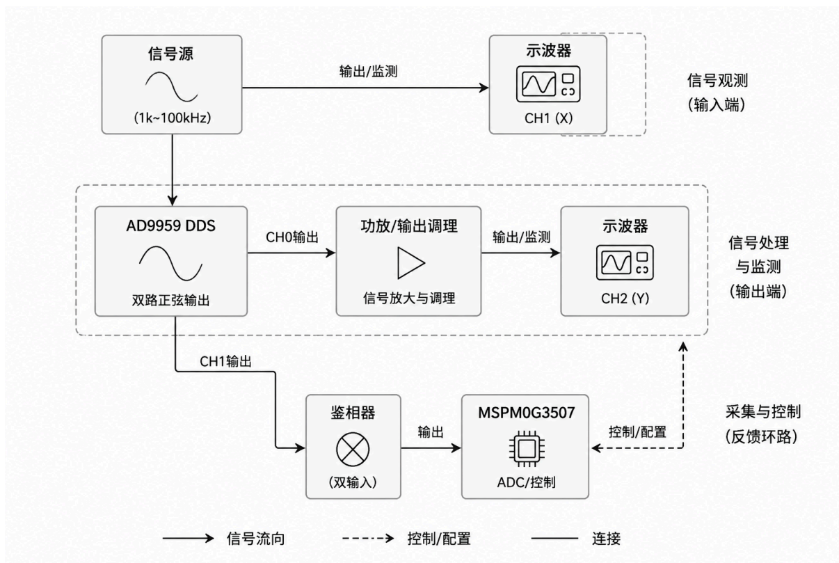
图 1 装置系统总体框图
