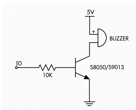
图 5 声光提示电路原理图
