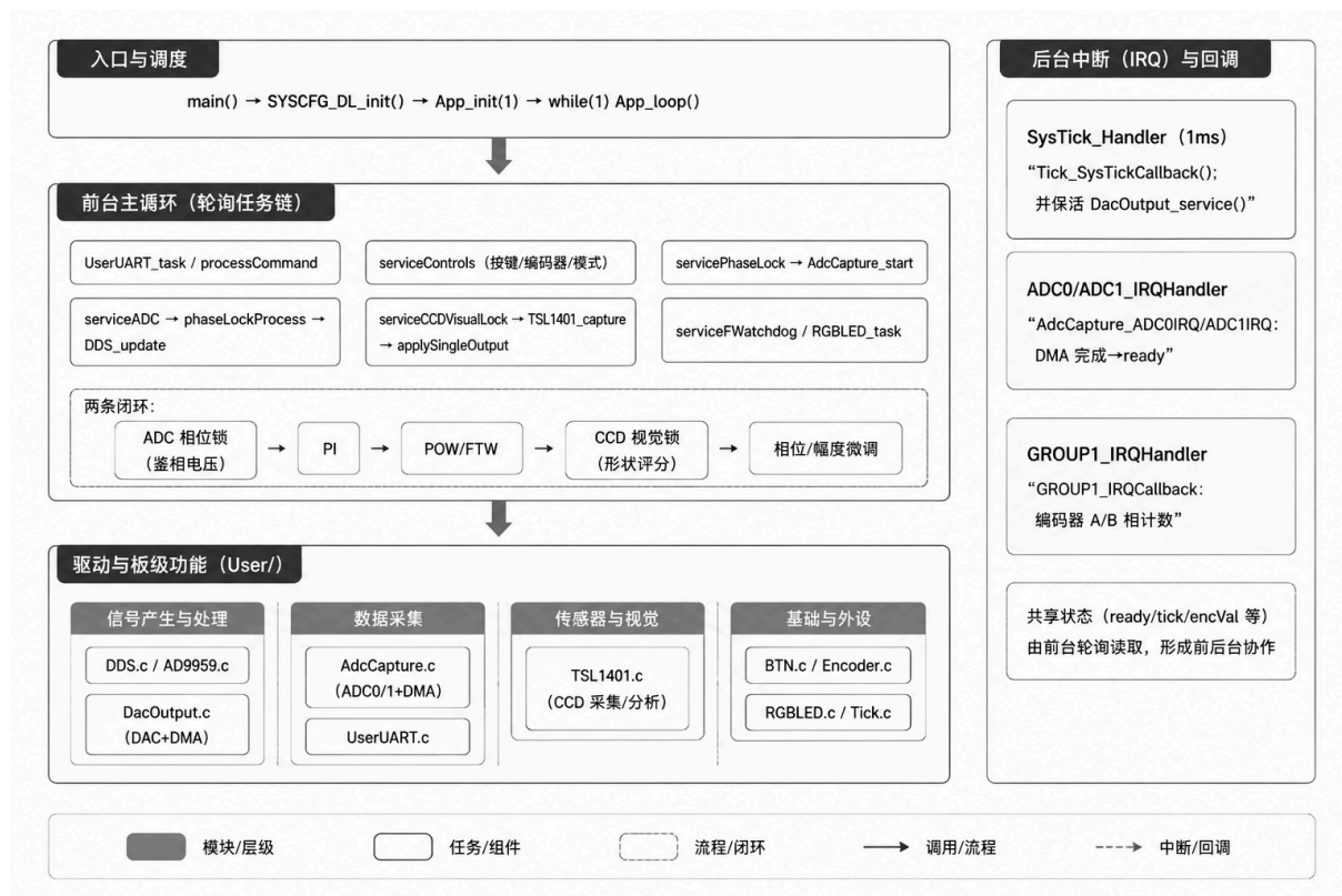
图 7 固件软件架构与前后台协作框图
