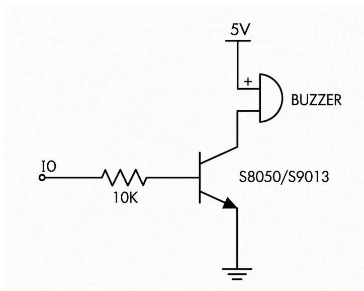
图 6 蜂鸣器与声光提示电路原理图
