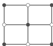
3 \times 3 网格图
