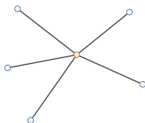
星形图 K_{1,5}
