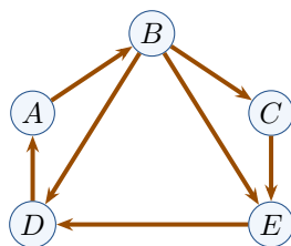
欧拉：看边
