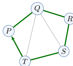
哈密顿：看点
