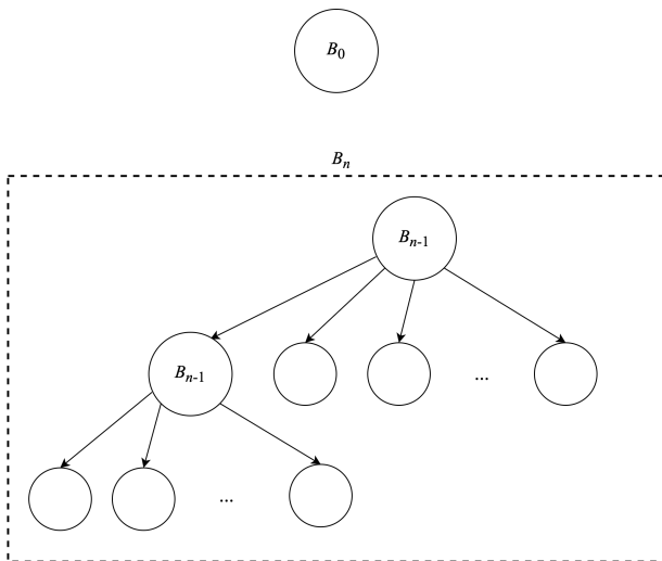
图 10.1: 二项式树
