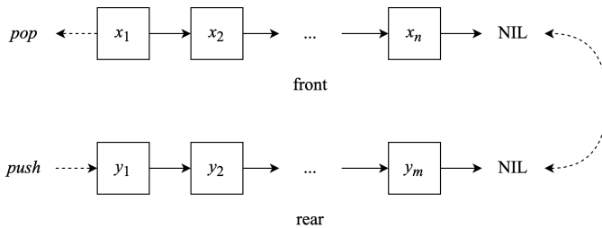
图 11.5: 双列表队列
