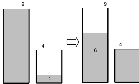
图 14.25: 最后两步
