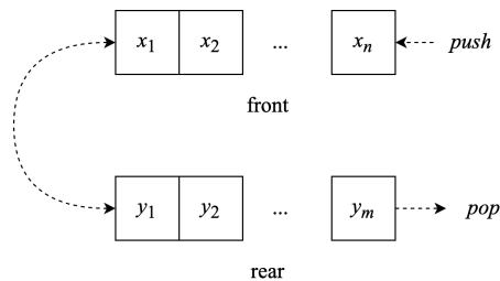
图 11.6: 双数组队列
