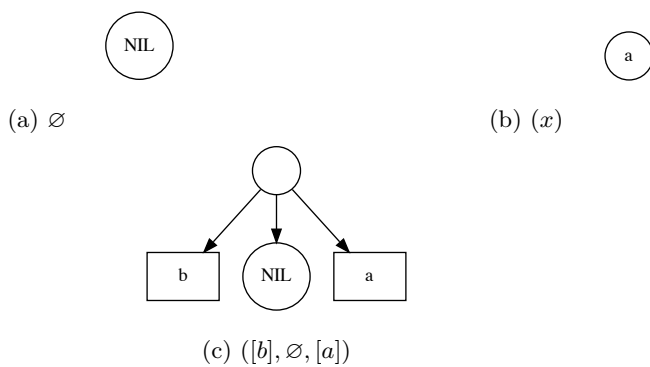
图 12.7: 手指树, 例 1
