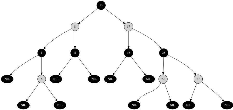
图 4.4: 红黑树
