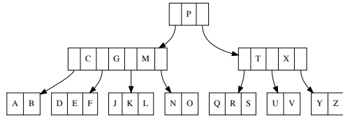
图 7.10: 删除前
