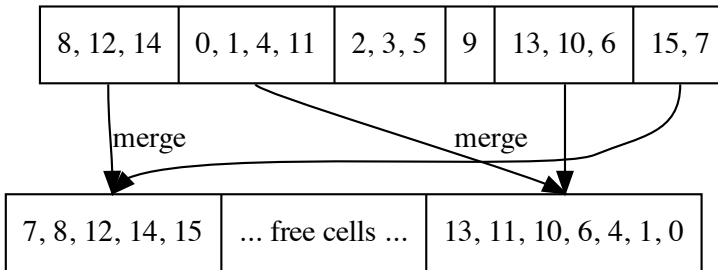
图 13.15: 自然归并排序
