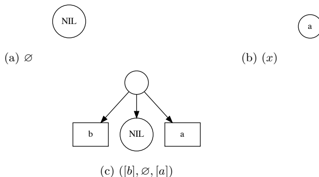
图 12.7: 手指树, 例 1
