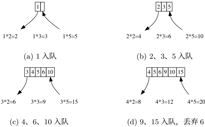
图 2: 前 4 步
