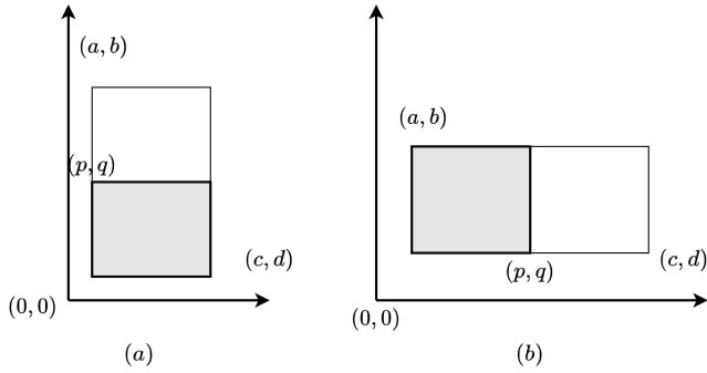
图 14.10: 沿中线二分查找时的特殊情况
