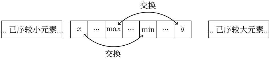
图 9.4: 一次扫描同时定位出最小和最大元素, 然后将它们放到正确的位置
