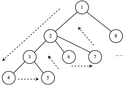
图 14.21: 深度优先搜索的顺序
