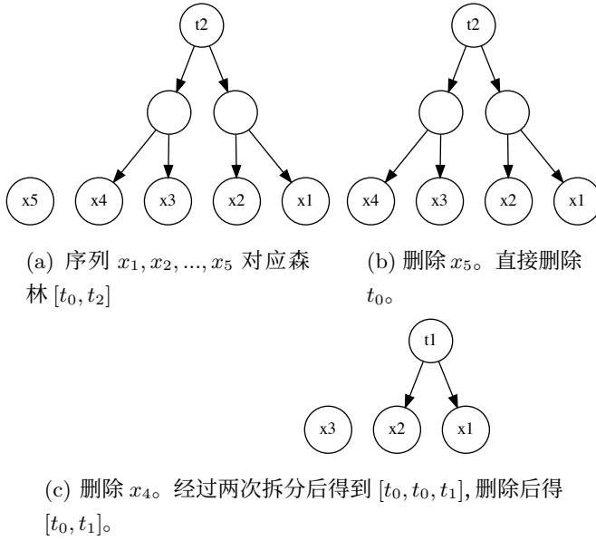
图 12.3: 从头部删除元素
