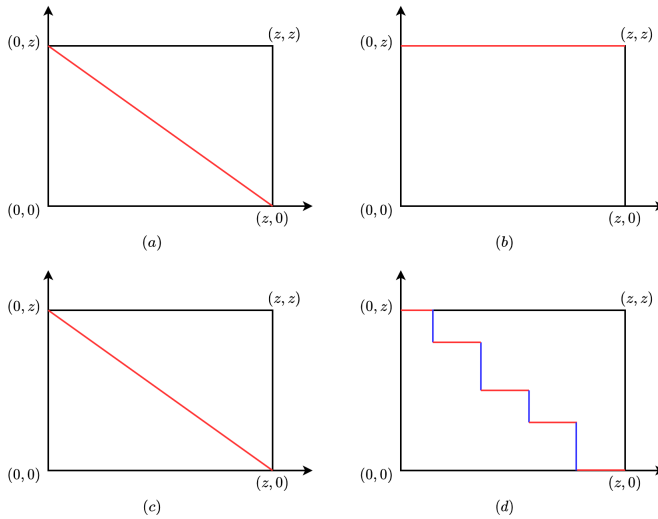
图 14.4: 最好和最差情况
