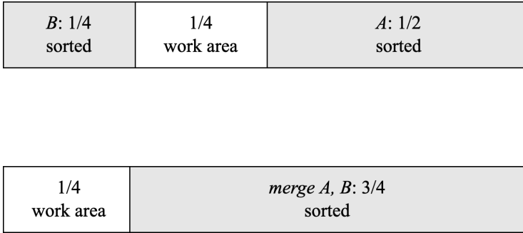
图 13.13: 利用工作区归并 A、B
