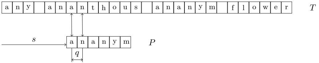
(b) 偏移到 s = 4 + 2 = 6 。
