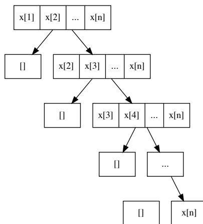
(a) [x_1 < x_2 < \dots < x_n] 的划分树。≤ p 的部分总为空。
