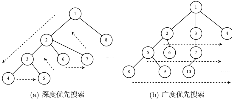
图 14.31: 深度和广度优先搜索的顺序
