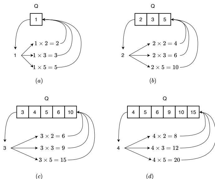
图 2: 前 4 步: 1 入队; 2、3、5 入队; 4、6、10 入队; 9、15 入队, 丢弃 6
