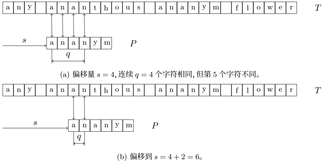
图 14.12: 在文本“any ananthous any m flower”中寻找“anany m”
