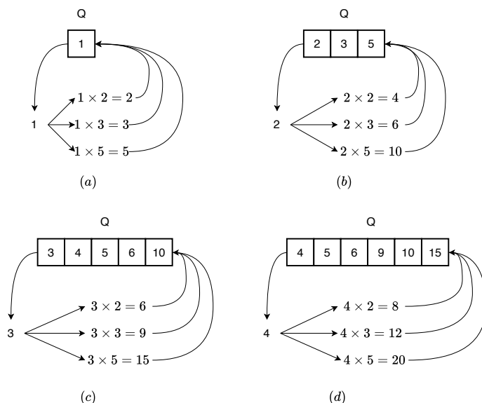
图 2: 前 4 步: 1 入队; 2、3、5 入队; 4、6、10 入队; 9、15 入队, 丢弃 6
