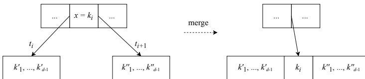
图 7.14: 先合并再删除
