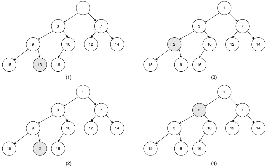
图 8.4: 将 13 减小为 2。2 先与 9 交换,然后再与 3 交换。
