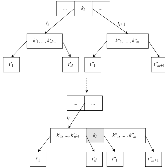
图 7.17: 合并 t_i 、 k 、 t_{i+1}
