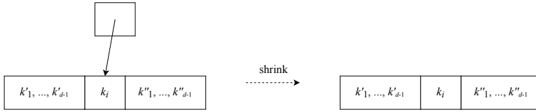
图 7.15: 缩减高度
