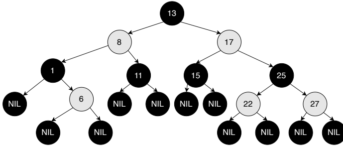
图 4.4: 红黑树
