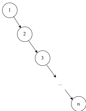
图 4.1: 不平衡的树
