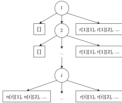
图 12.9: 不规则树, 第 i 层子树的 f 不为空
