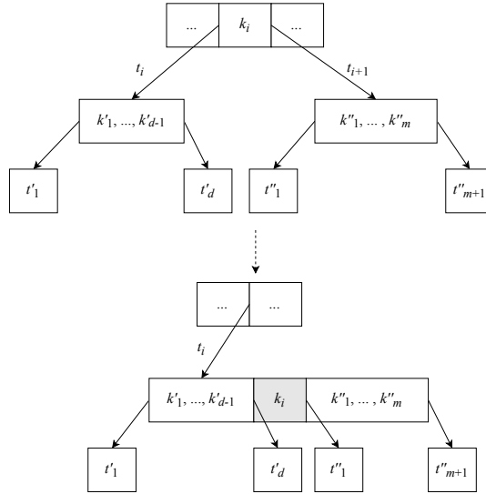
图 7.17: 合并 t_i 、 k 、 t_{i+1}
