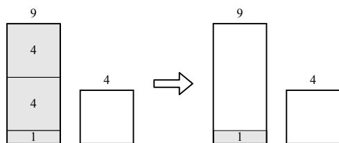
图 14.26: 将大瓶倒满, 然后倒入小瓶两次
