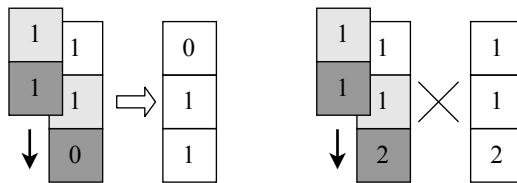
图 14.30: 左侧:两个标 1 的格子都可移动;右侧:下方标 1 的格子和标 2 的格子冲突。
