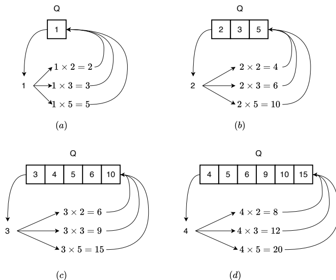
图 2: 前 4 步
