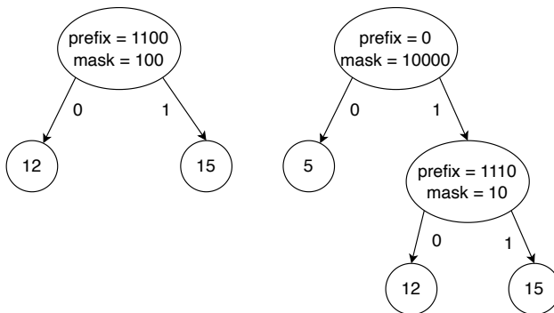
(b) 插入 5 = (101)_2 , 它和最长公共前缀 p = (1100)_2 不匹配, 分出一个新叶子节点。
