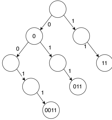
图 6.2: 大端(big-endian) trie
