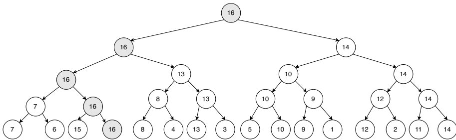
图 9.5: 元素 15 在第一轮就被淘汰
