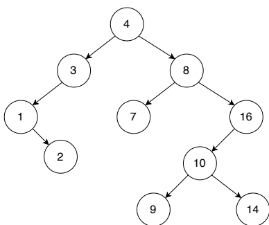
图 2.2: 二叉搜索树的例子
