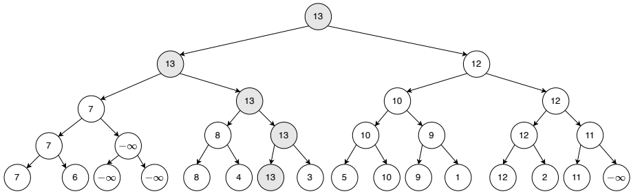
图 9.6: 锦标赛树排序的前几步
