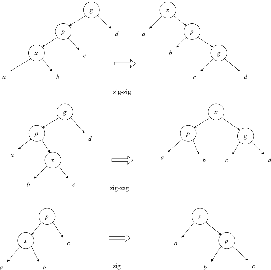
图 8.10: zig-zig: x 和 p 都是左子树或都是右子树, x 成为根节点。zig-zag: x 和 p 一棵是左子树另一棵是右子树, x 成为根节点, p 和 g 变成了兄弟节点。zig: p 是根节点, 旋转后 x 变为根节点。
