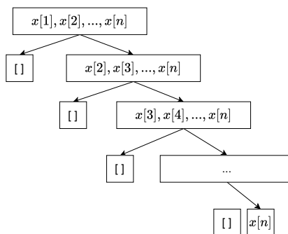
(a) [x_1 < x_2 < \dots < x_n] 的划分树。 \leq p 的部分总为空。
