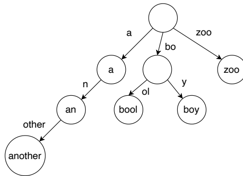
图 6.9: 一棵前缀树, 包含键: a, an, another, bool, boy, zoo
