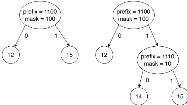
(a) 插入 14 = (1110)_2 , 它和最长公共前缀 p = (1100)_2 匹配, 递归插入右子树。
