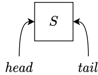
图 11.1: 空队列, 头、尾都指向 S
