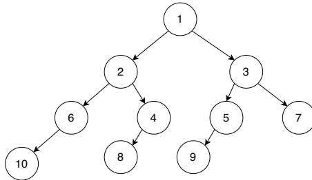
图 8.9: 用已序序列 [1, 2, ..., 10] 构造的斜树
