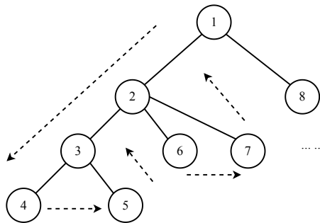
图 14.21: 深度优先搜索的顺序
