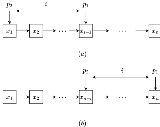
图 1.2: 双指针滑动窗口。(a) p_2 指向表头, 距离 p_1 之后 i 步; (b) 当 p_1 到达表尾时, p_2 指向右数第 i 个。
