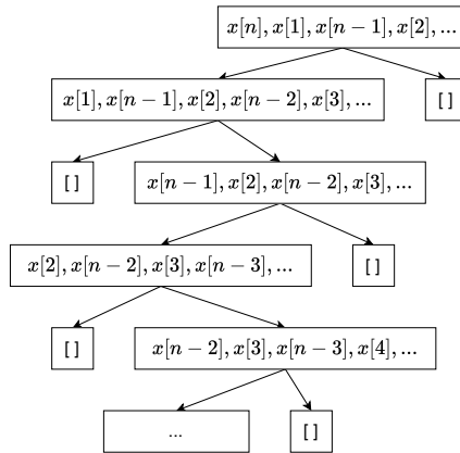
(b) 一个之字形的划分树。
