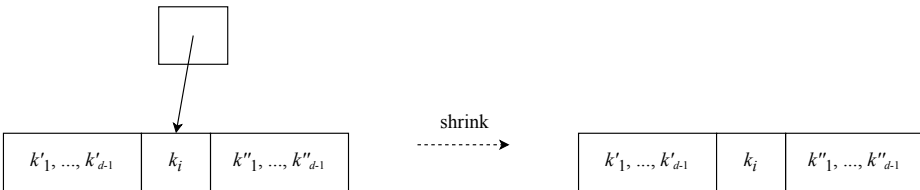
图 7.15: 缩减高度
