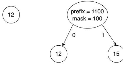
图 6.5: 左: T 是叶子节点 12; 右: 插入 15 后
