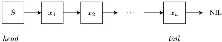
图 11.2: 带有 S 节点的列表
