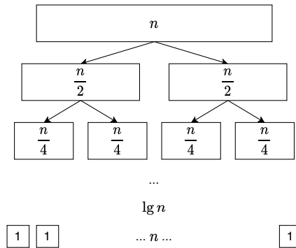
图 13.2: 最好情况,每次均分。
