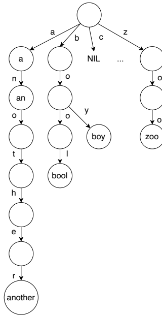
图 6.8: 含有多达 26 个分枝的 trie, 包含键: a、an、another、bool、boy、zoo
