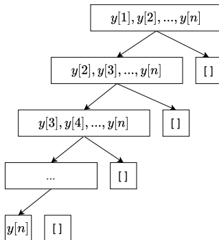
(b) [y_1 > y_2 > \dots > y_n] 的划分树， \geq p 的部分总为空。
