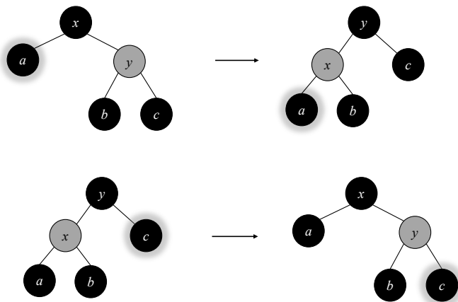
图 38: 双重黑色节点的兄弟节点为红色
