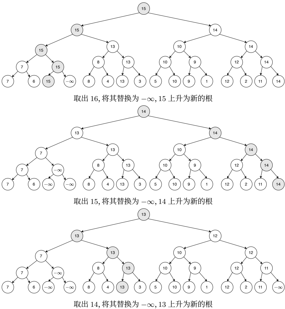
图 9.6: 锦标赛树排序的前几步
