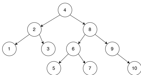
图 5.1: AVL 树
