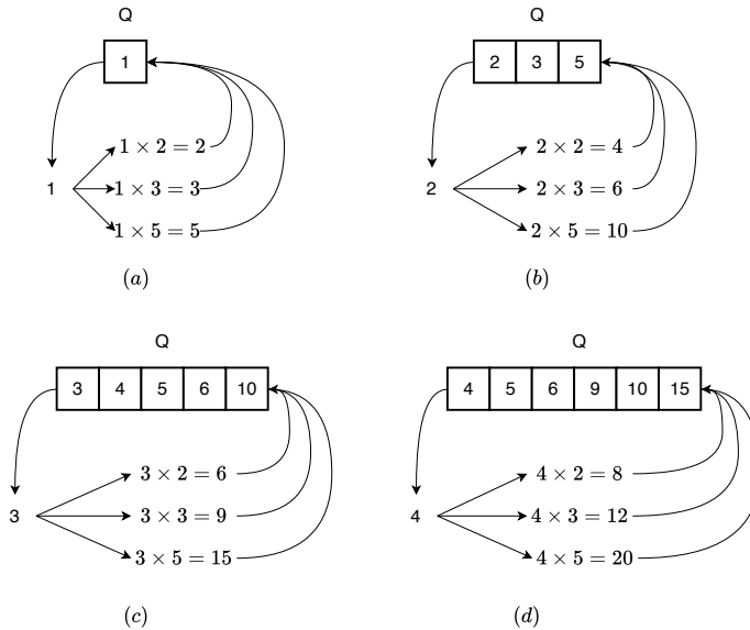
图 2: 前 4 步
