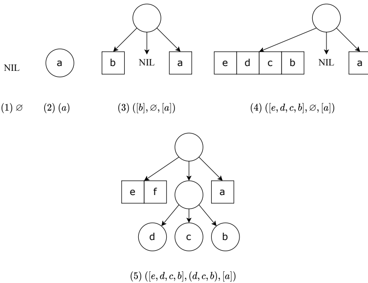
图 12.7: 手指树
