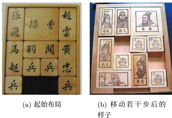
图 14.28: 华容道游戏
