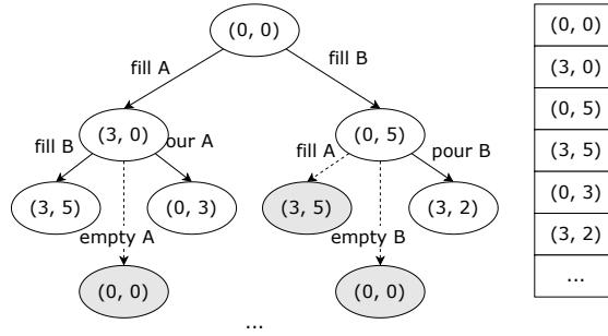
图 14.27: 全局记录
