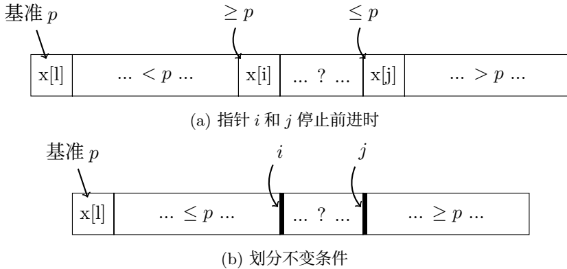
图 13.3: 双向扫描
