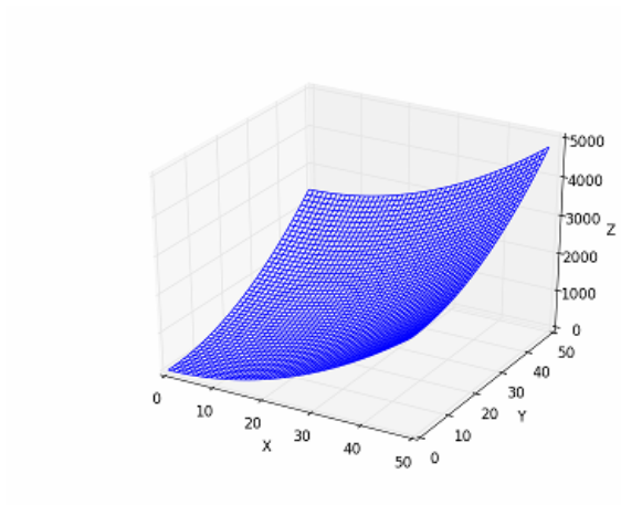
图 14.5: f(x, y) = x^2 + y^2 的图像
