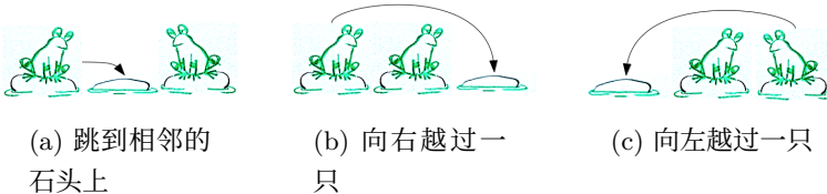
图 14.19: 移动规则
