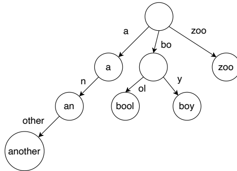
图 6.9: 一棵前缀树, 包含键: a, an, another, bool, boy, zoo
