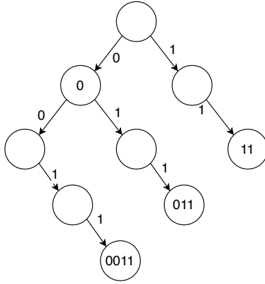
图 6.2: 大端(big-endian)trie
