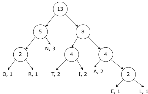
图 14.34: 哈夫曼树
