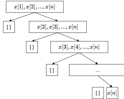
(a) [x_1 < x_2 < \dots < x_n] 的划分树。≤ p 的部分总为空。
