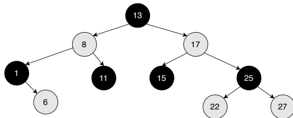
图 4.5: 隐藏 NIL 节点
