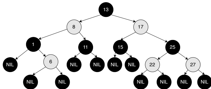
图 4.4: 红黑树
