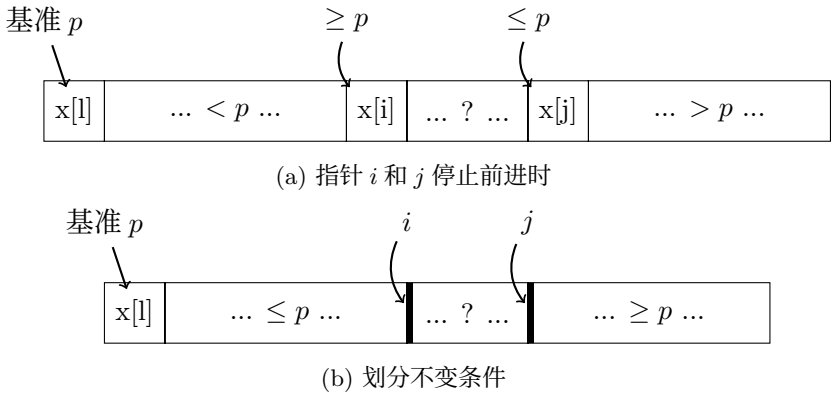
图 13.3: 双向扫描
