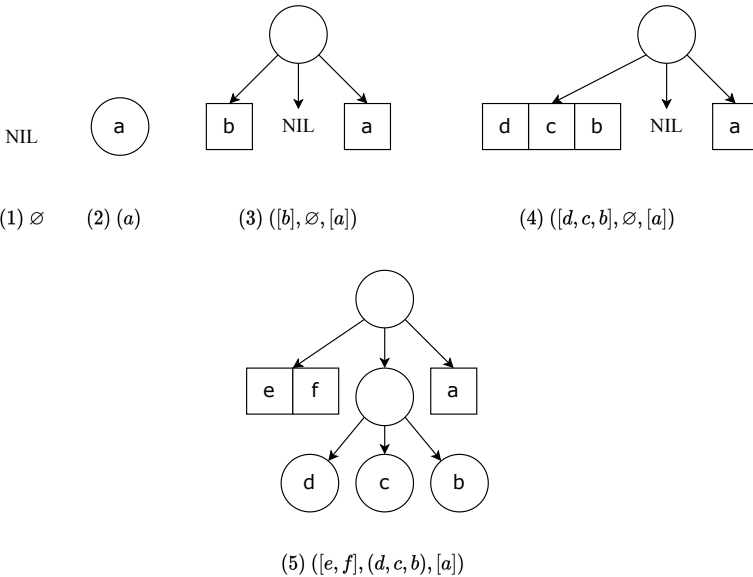
图 12.7: 手指树
