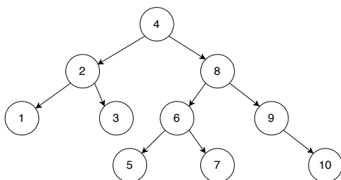
图 5.1: AVL 树
