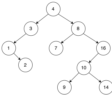
图 2.3: 8 的后继为其右侧分支的最小值 9; 为了获得 2 的后继, 首先向上找到 1, 它没有左子树, 继续向上找到 3, 3 的左子树也是 2 的祖先, 故而后继为 3。
