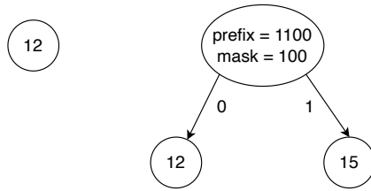
图 6.5: 左: T 是叶子节点 12; 右: 插入 15 后
