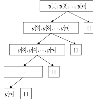
(b) [y_1 > y_2 > \dots > y_n] 的划分树, \geq p 的部分总为空。
