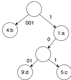
图 6.4: 小端整数树实现的映射 \{1 \rightarrow a, 4 \rightarrow b, 5 \rightarrow c, 9 \rightarrow d\}
