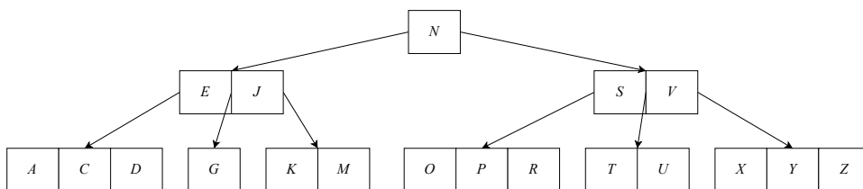
图 7.1: B 树
