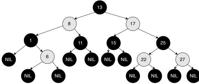
图 4.4: 红黑树
