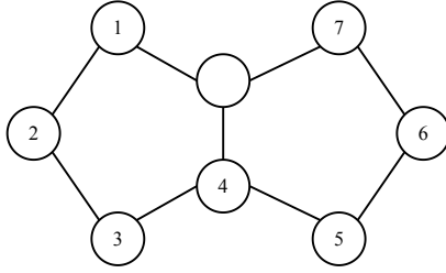
图 14.33: 康威滑动趣题
