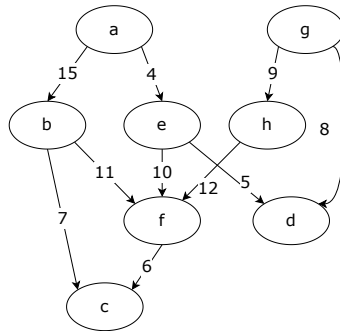
图 14.32: 带权重的有向图
