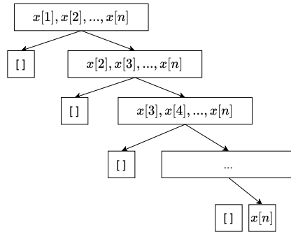
(a) [x_1 < x_2 < \dots < x_n] 的划分树, \leq p 的部分总为空。
