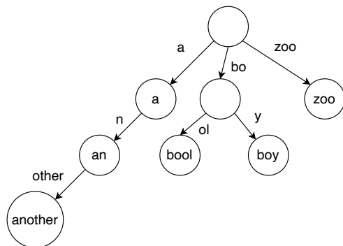
图 6.9: 一棵前缀树, 包含键: a、an、another、bool、boy、zoo
