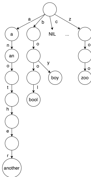
图 6.8: 含有多达 26 个分枝的 trie, 包含键: a、an、another、bool、boy、zoo
