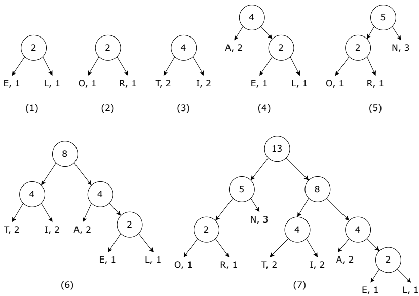
图 14.35: 构造哈夫曼树
