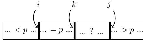
图 13.5: 单向扫描三路划分
