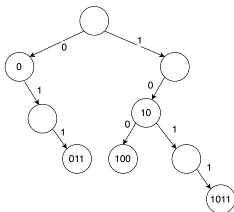
图 6.1: 基数树
