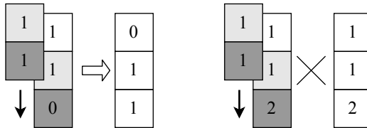
图 14.30: 左侧:两个标 1 的格子都可移动;右侧:下方标 1 的格子 and 标 2 的格子冲突。
