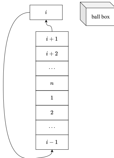
图 14.23: 第 i 个人出队摸球。如果没有摸到黑球就站到队尾。
