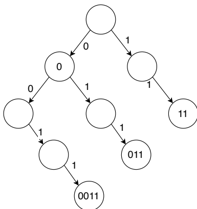
图 6.2: 大端(big-endian)trie
