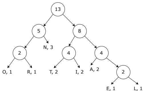
图 14.34: 哈夫曼树
