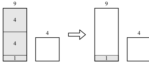
图 14.26: 将大瓶倒满, 然后倒入小瓶两次
