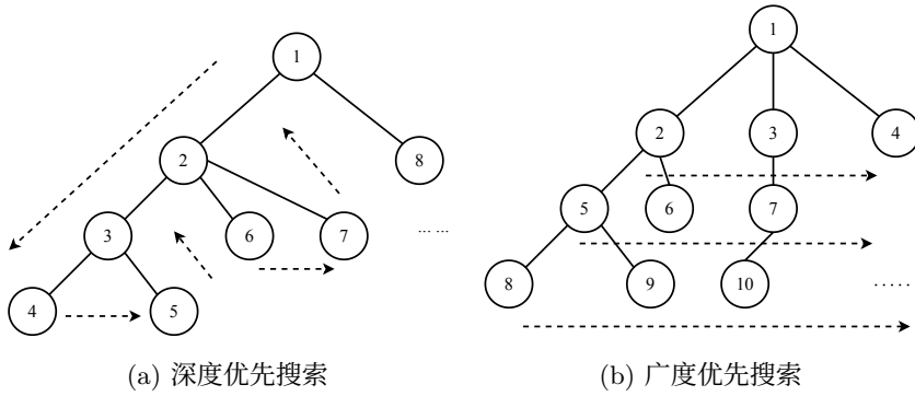
图 14.31: 深度和广度优先搜索的顺序
