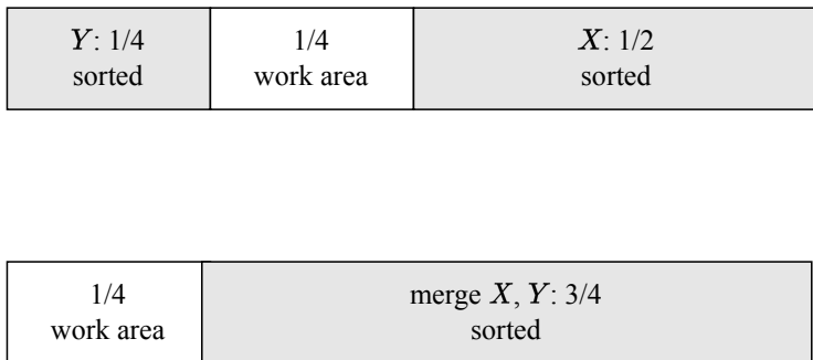
图 13.13: 利用工作区归并 X 、 Y
