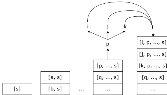
图 14.16: 用栈记录路径
