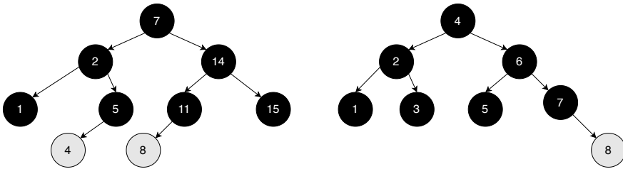
图 4.7: 插入产生的红黑树
