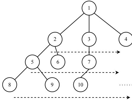
图 14.24: 从第一个状态开始, 检查第二步的所有选项 2、3、4; 然后检查第 3 层上的所有选项.....
