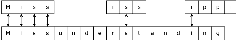
图 14.36: 最长公共子序列
