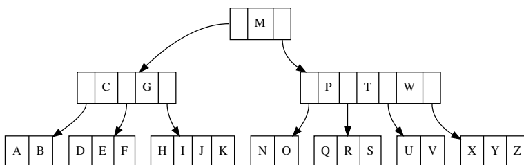
图 7.1: B 树
