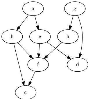
图 14.34: 一个有向图
