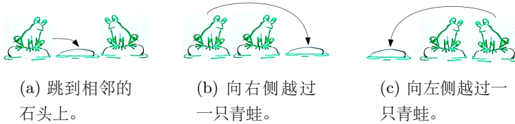
图 14.31: 移动规则
