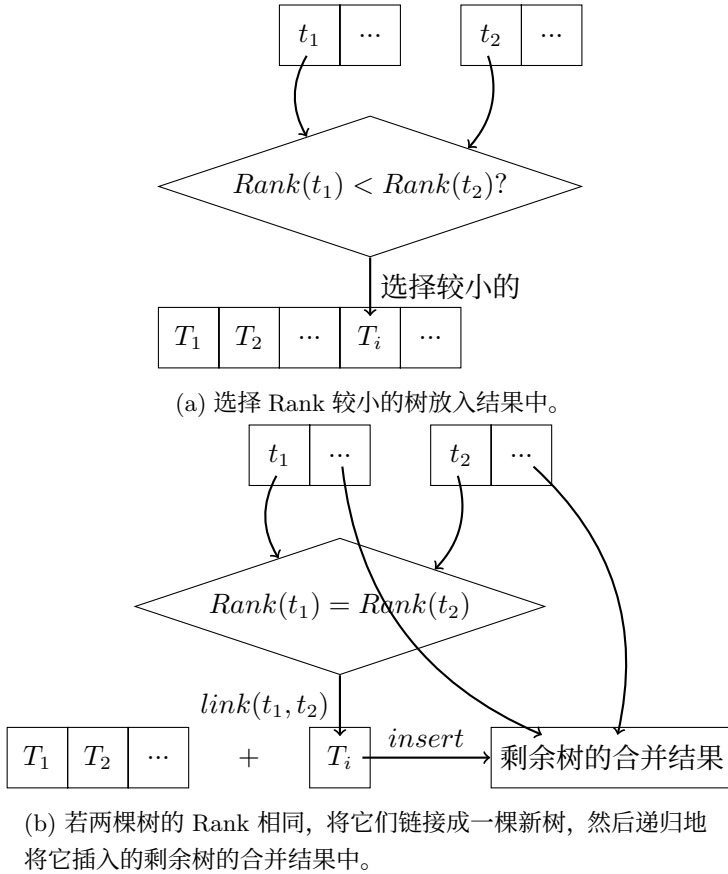
图 10.7: 堆合并
