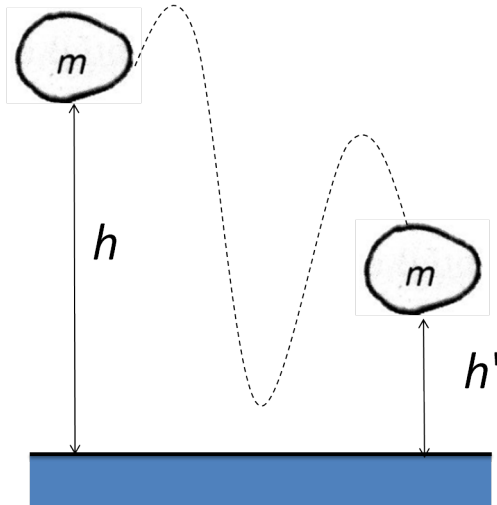
图 10.11: 重力势能
