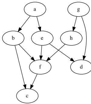
图 14.34: 一个有向图
