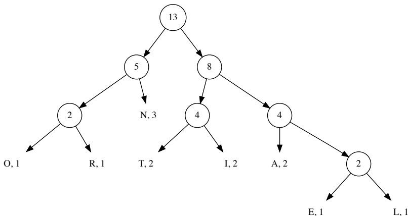
图 14.47: 一棵编码树
