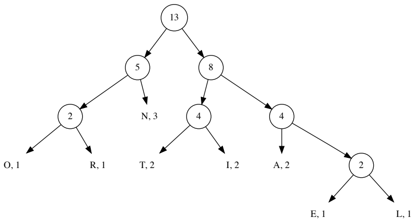
图 14.47: 一棵编码树
