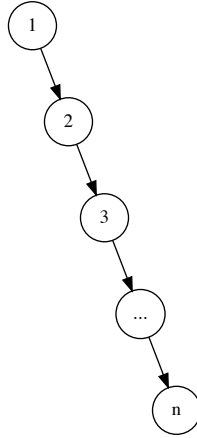
图 4.1: 不平衡的树
