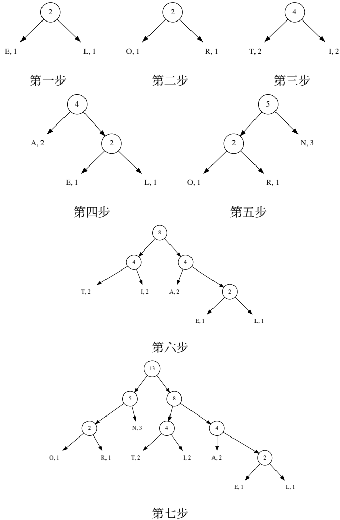
图 14.48: 构造一棵 Huffman 树的步骤
