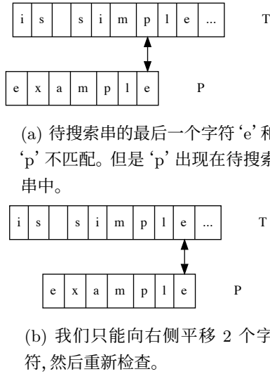
图 14.19: 如果不匹配的字符出现在待搜索串中, 需要向右侧少量平移
