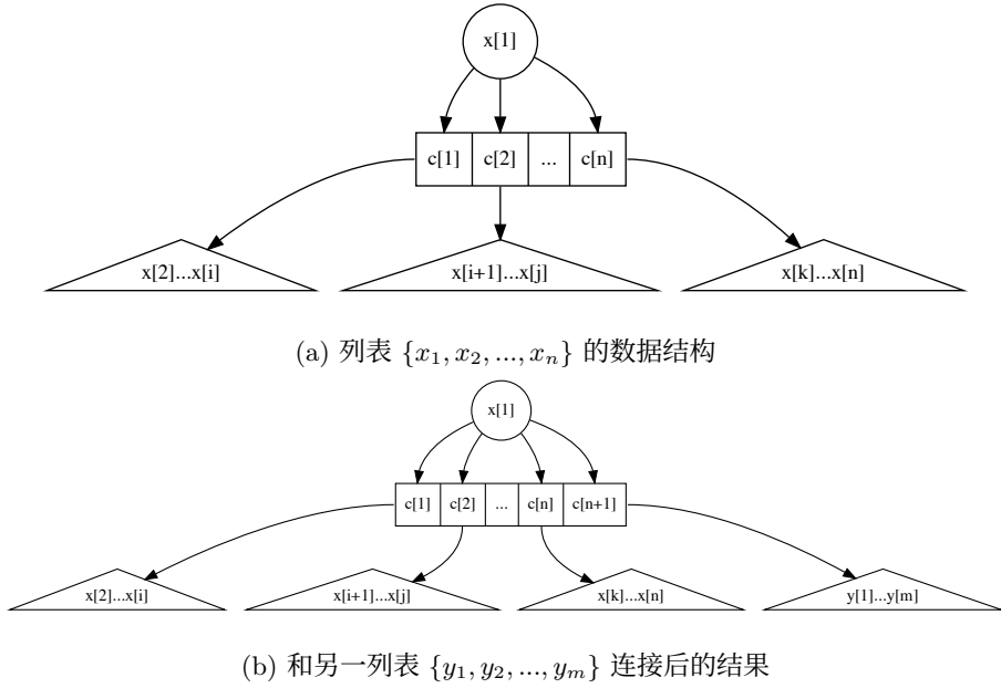
图 12.6: 可连接列表的数据结构
