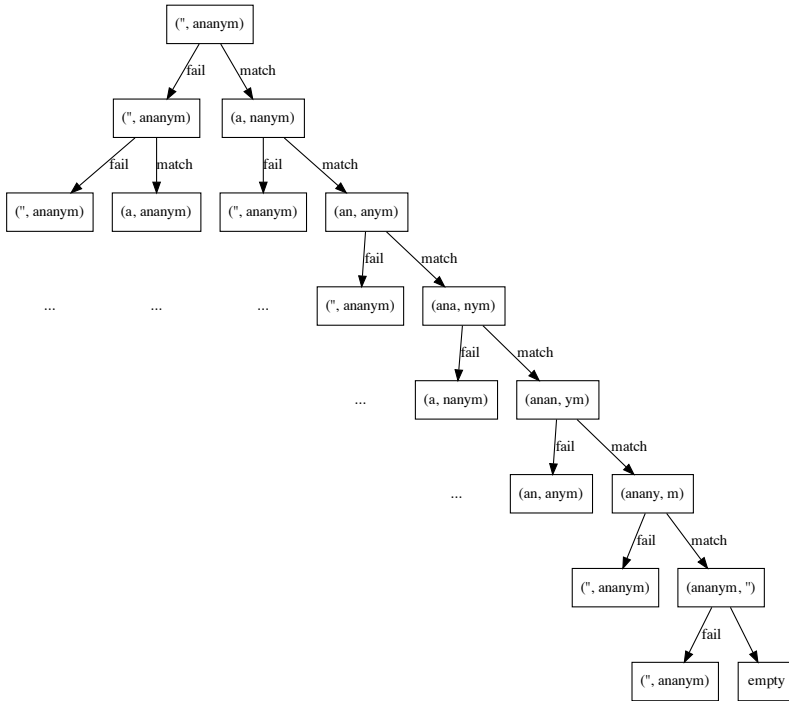
图 14.16: 从字符串“anonym”构造的无穷状态树
