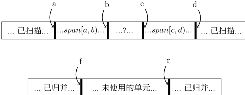
图 13.18: 自然归并排序时的不变性质
