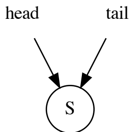
图 11.1: 空队列,头部和尾部都指向 sentinel 节点
