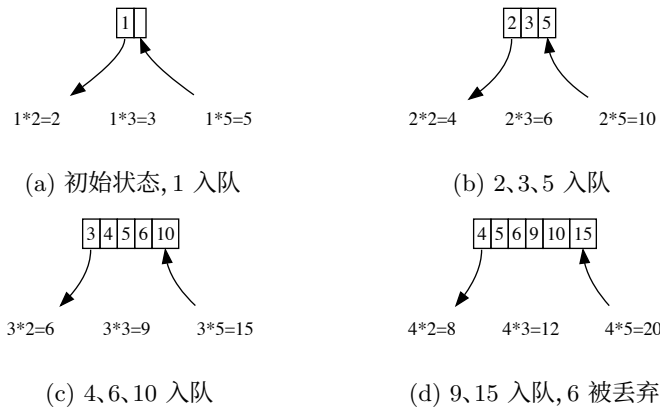
图 2: 使用队列生成正规数的前 4 步
