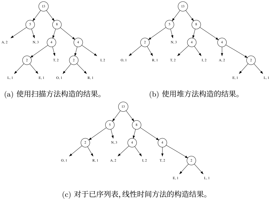
图 14.49: 同样的字符列表构造出的不同 Huffman 树
