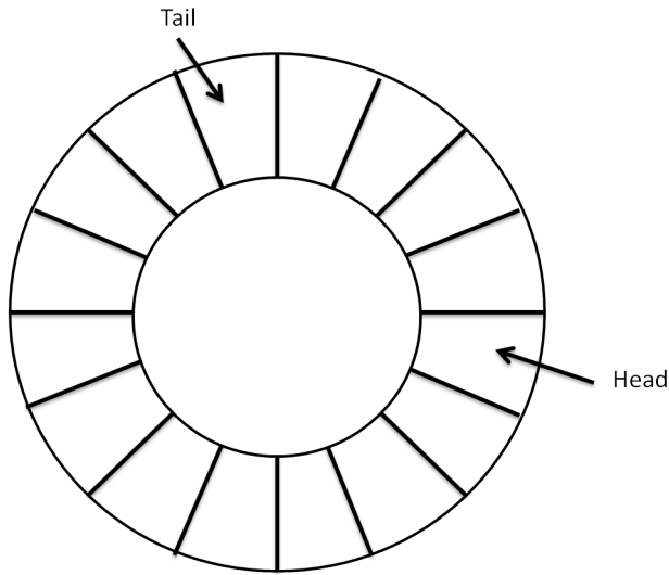
图 11.4: 循环缓冲区
