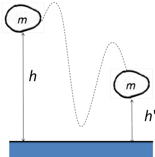
图 10.11: 重力势能
