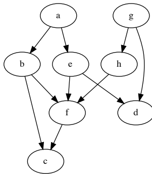
图 14.34: 一个有向图
