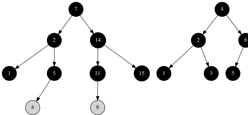
图 4.7: 插入产生的红黑树
