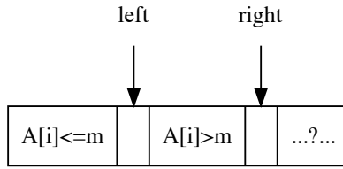
图 1: 数组划分。位于 0 \leq i < left 的元素满足 A[i] \leq m , 位于 left \leq i < right 的元素满足 A[i] > m , 剩余的元素尚未处理。
