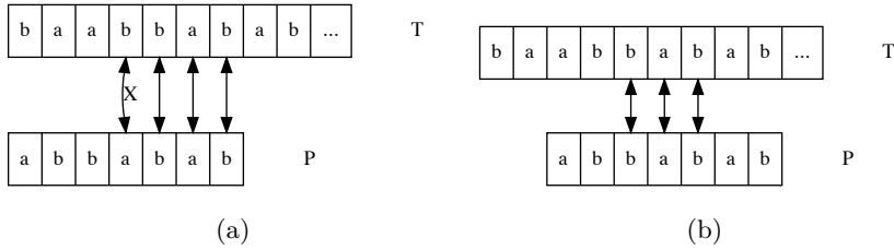
图 14.23: 已匹配的部分“bab”也在待搜索串的其他位置出现(从第 3 个字符到第 5 个字符)。我们只能向右平移 2 个单位以避免漏掉可能的解。
