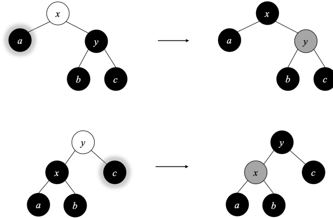
图 A.3: 向上传递黑色
