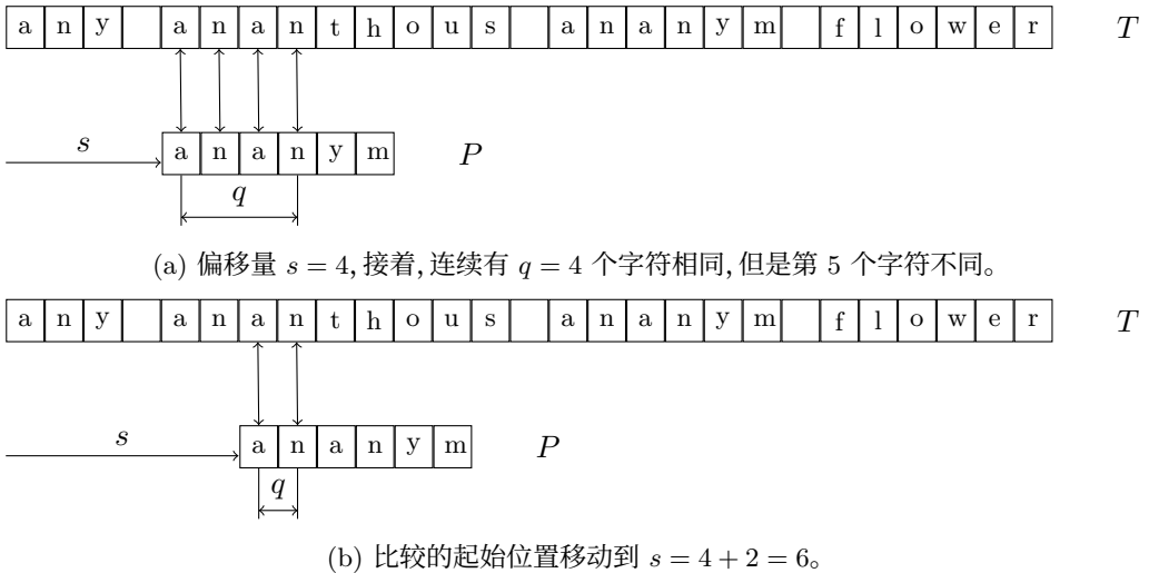
图 14.12: 在文本“any ananthous anany flower”中寻找“anany”
