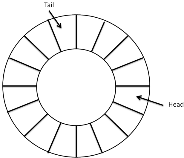
图 11.4: 循环缓冲区
