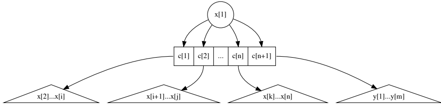
(a) 列表 \{x_1, x_2, \dots, x_n\} 的数据结构
