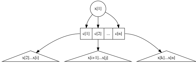
(a) 列表 \{x_1, x_2, \dots, x_n\} 的数据结构
