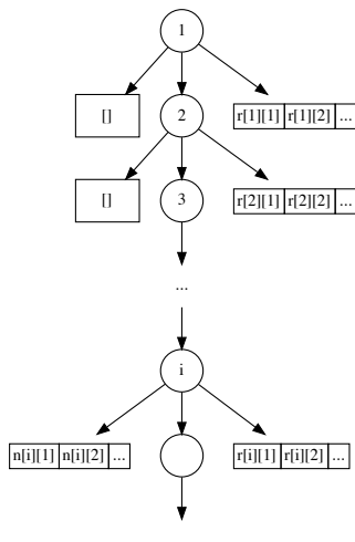
图 12.10: 不规则树的例子, 第 i 层子树的 front 手指不为空
