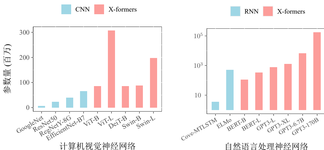
图 1.3: 神经网络参数量对比 Figure 1.3: Comparison of Neural Network Parameter Amount
