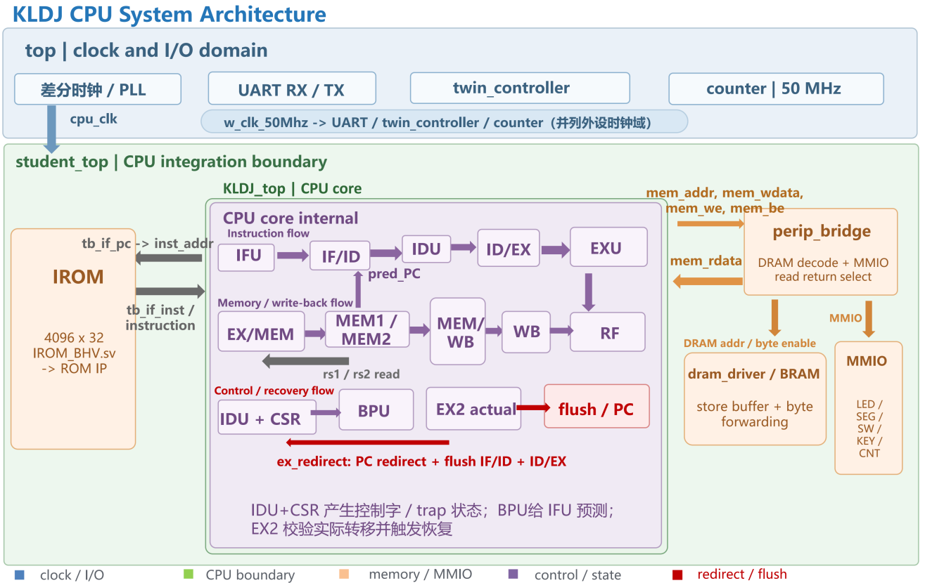
图 2.1 RISC-V 流水线 CPU、存储器与外设集成架构
