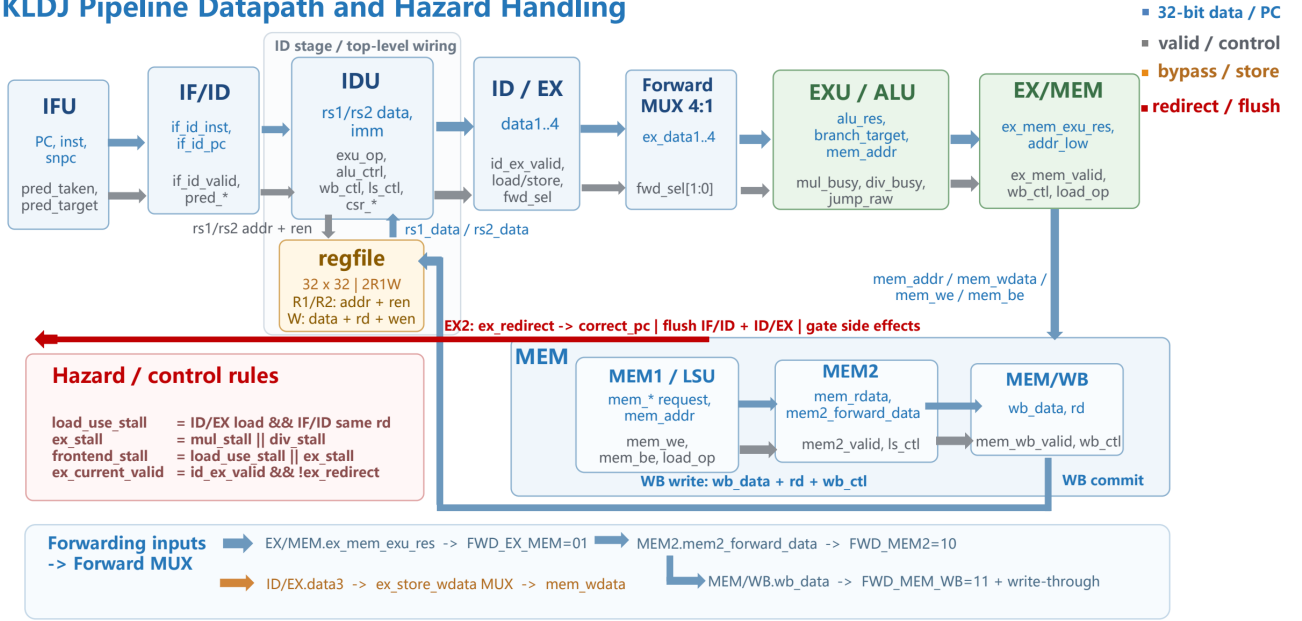
图 5.1 流水线冒险的检测与处理机制
