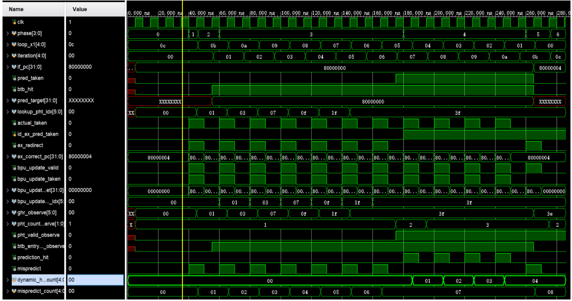
图 8.2 gshare、PHT 与 BTB 联合预测功能仿真
