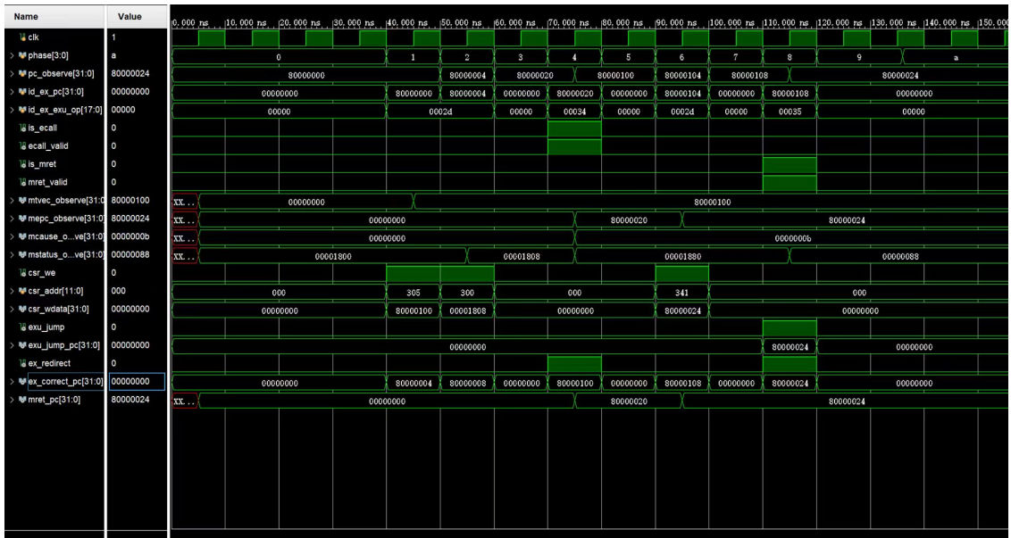
图 8.3 ecall 进入与 mret 返回功能仿真
