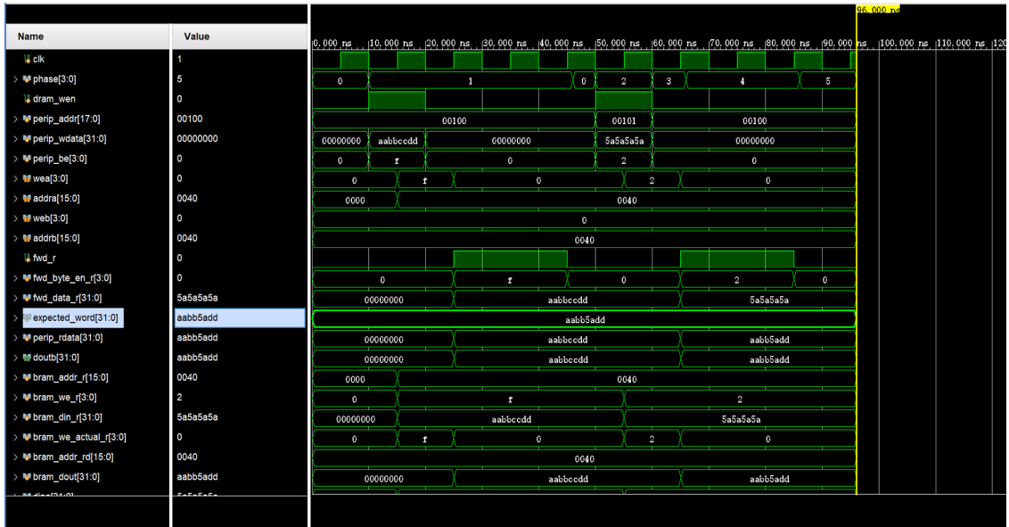
图 8.1 双端口 BRAM 及写后读前递功能仿真
