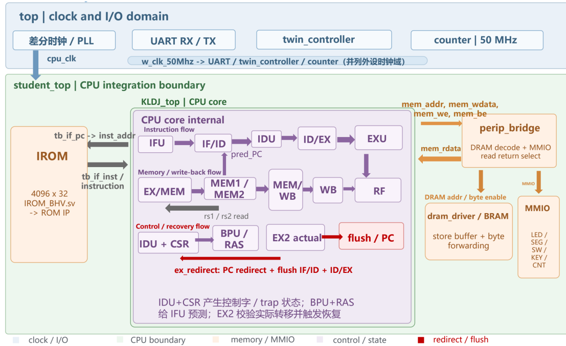
图 2.1 RISC-V 流水线 CPU 总体架构图
