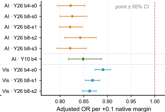
(d) Margin \rightarrow false negative (FN)
