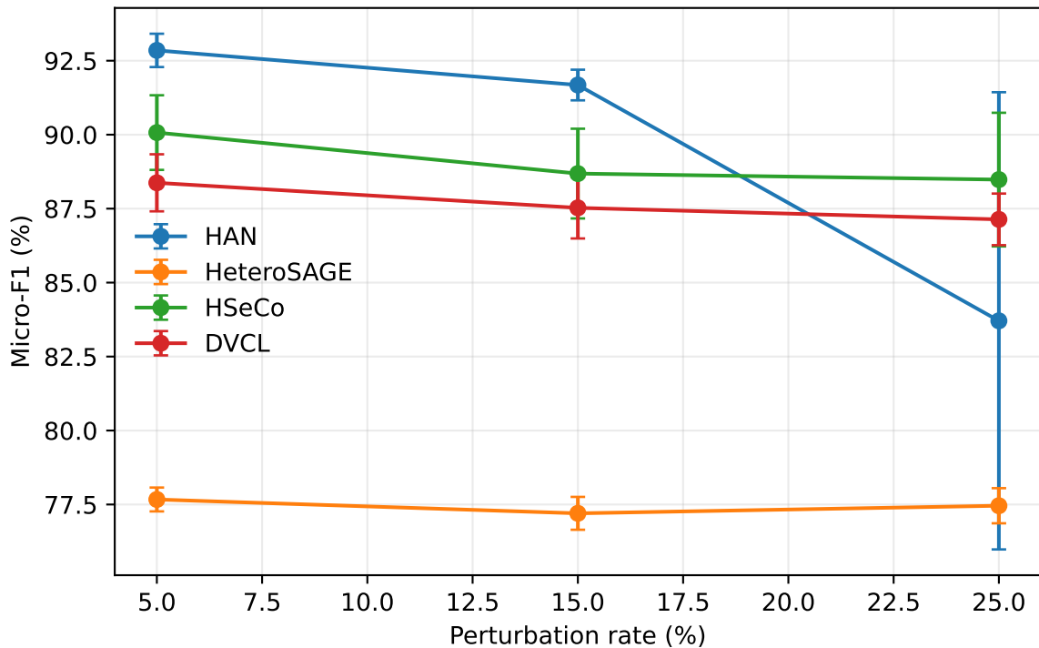
DBLP — PRBCD
