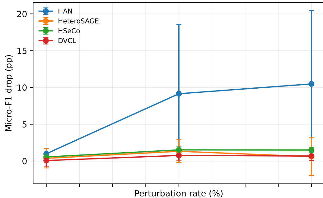
DBLP — HETEPRBCD
