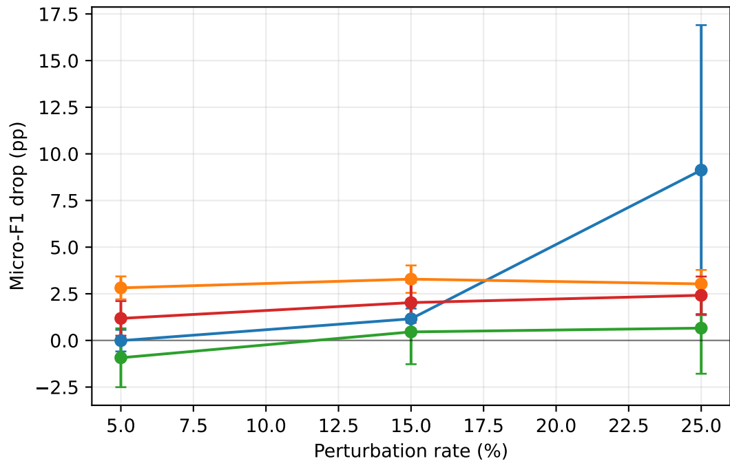
DBLP — PRBCD
