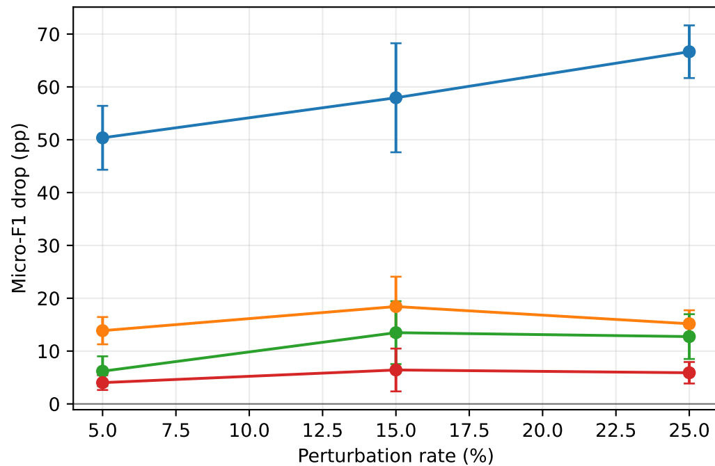
DBLP — HETEPRBCD
