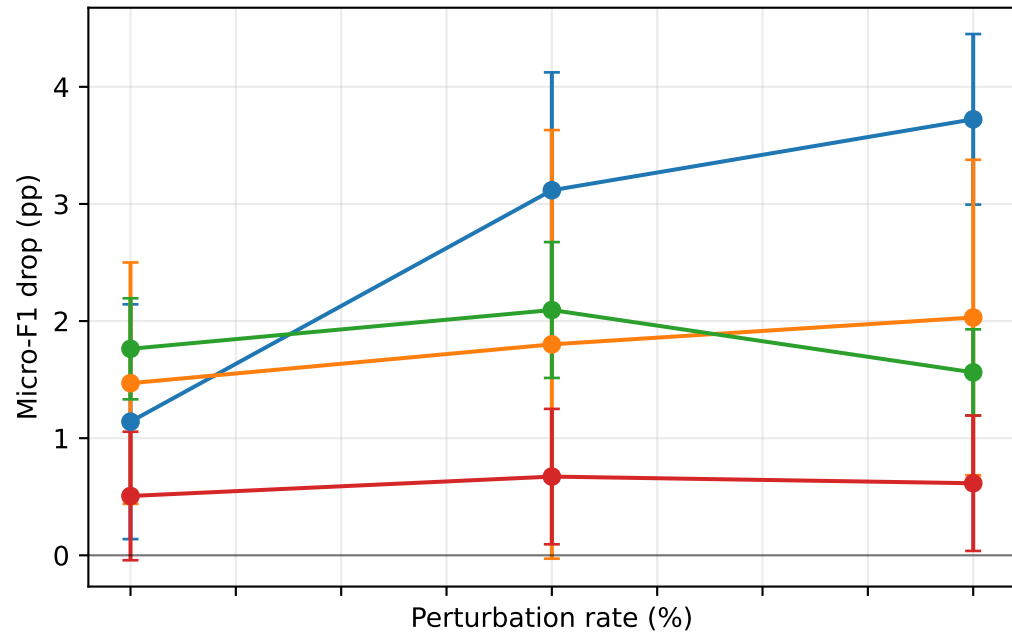
DBLP — PRBCD
